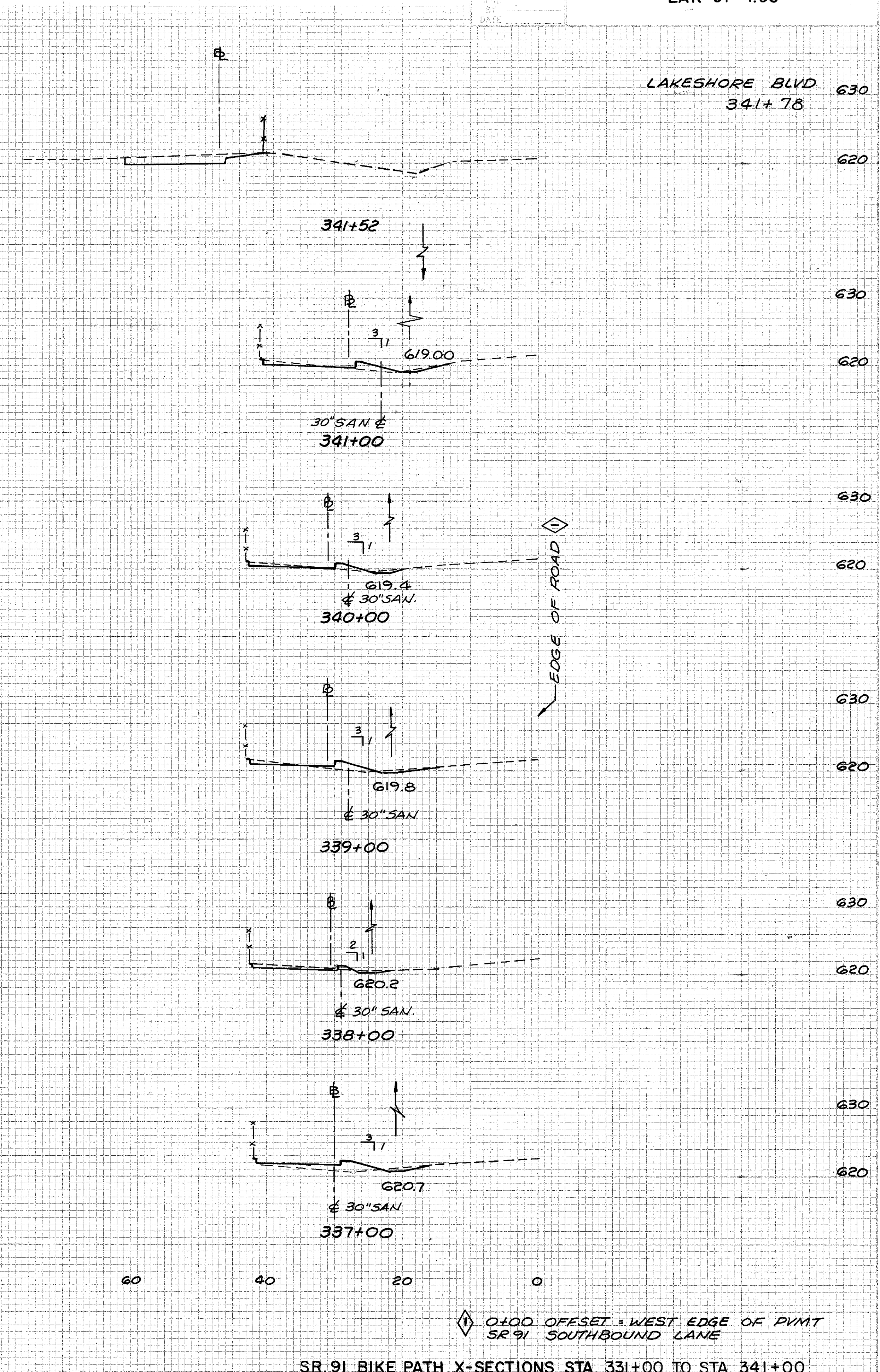
SR. 91 BIKE PATH X-SECTIONS STA. 331+00 TO STA. 341+00
