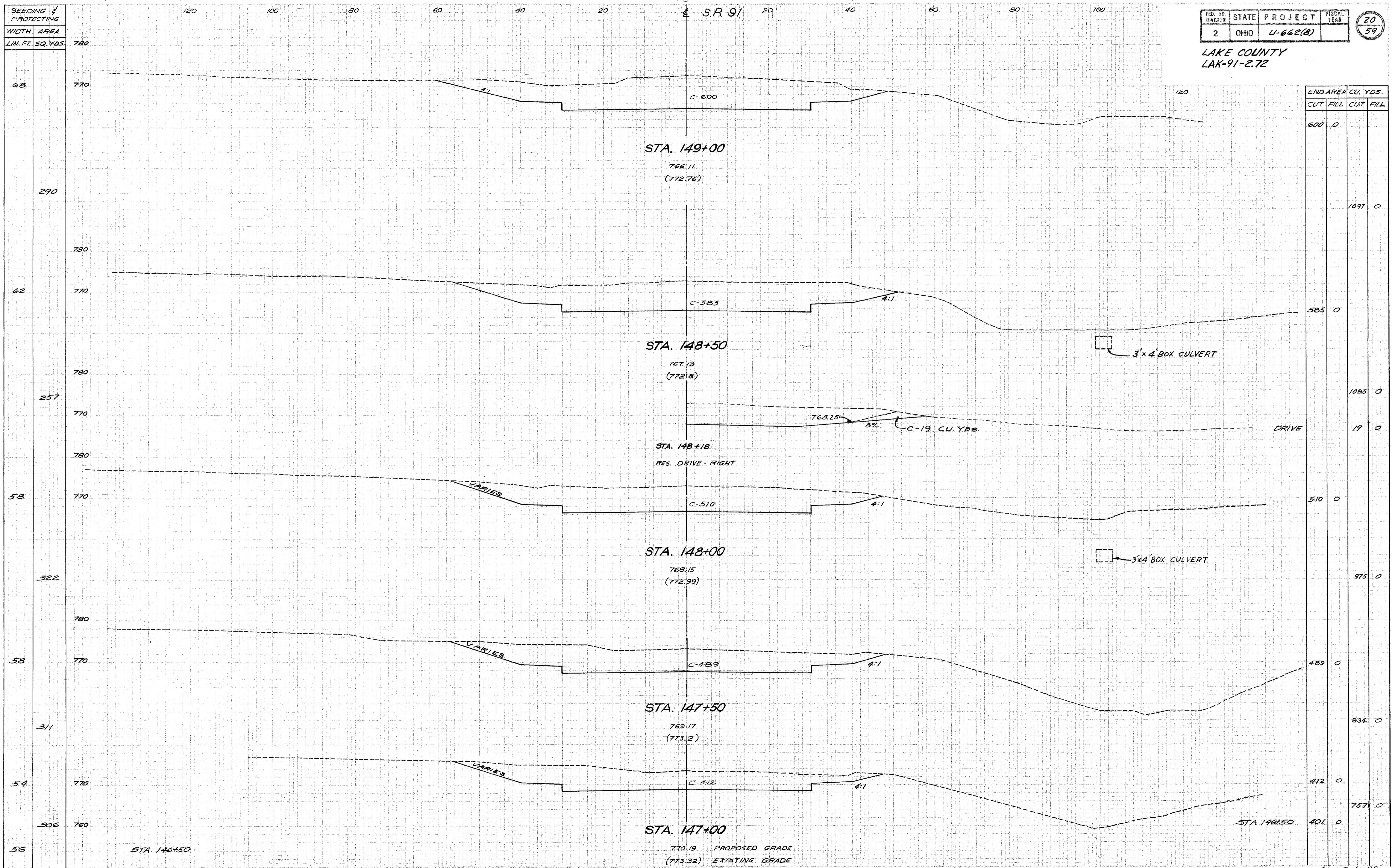
CROSS SECTIONS STA. 147+00 TO STA. 149+00
