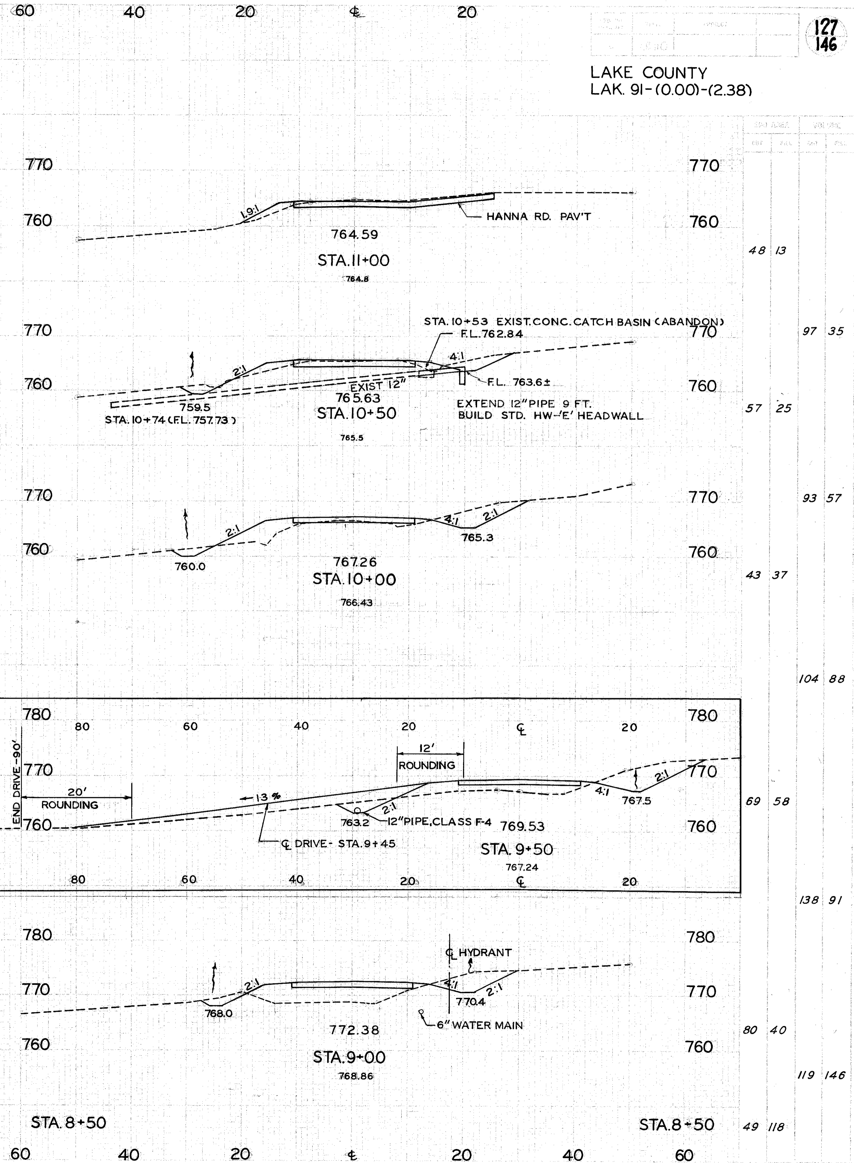
CROSS SECTION... MAPLE GROVE RD... STA. 6+50 TO STA. 11+00
