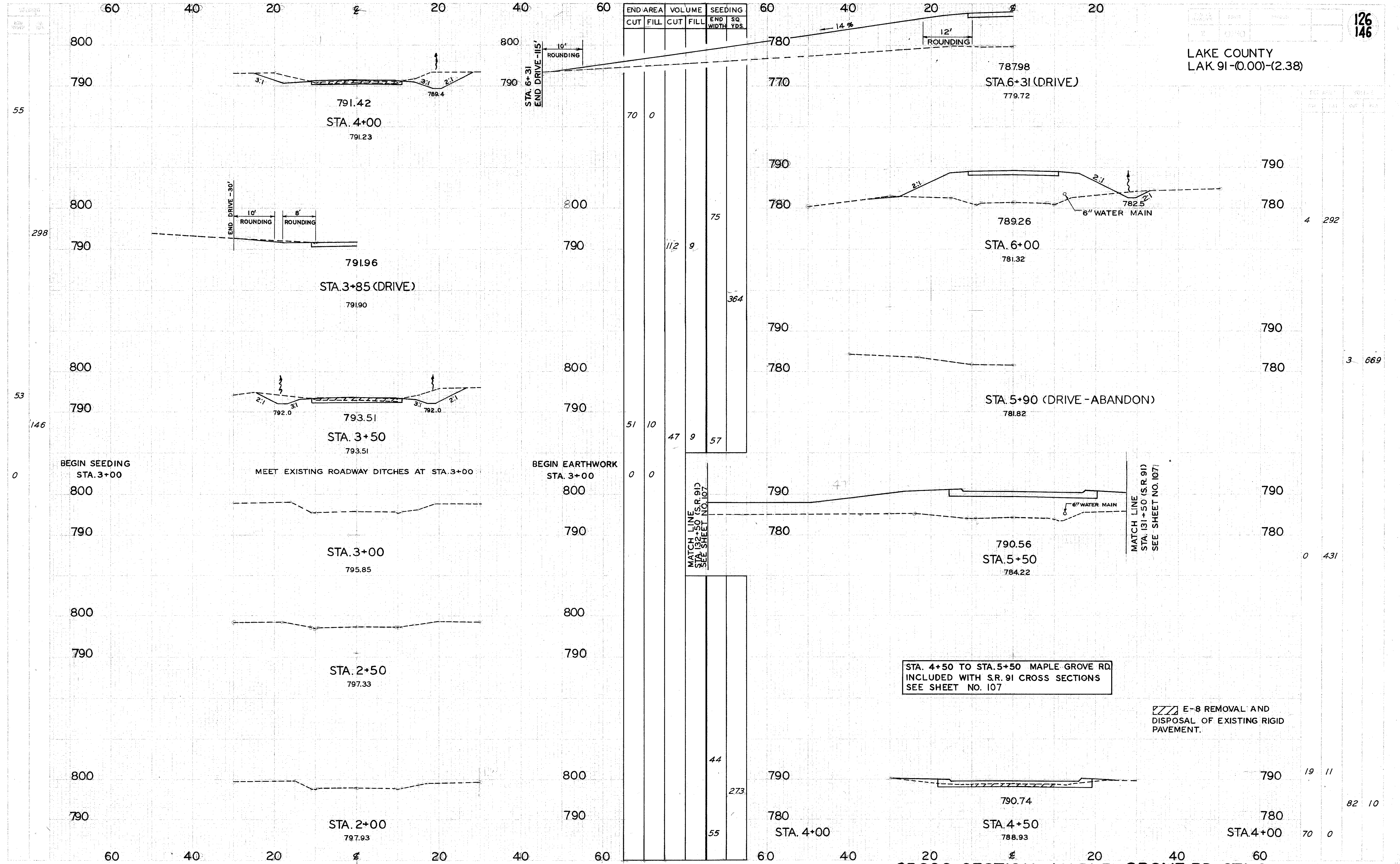
CROSS SECTION MAPLE GROVE RD STA. 2+00 TO STA. 6+31
