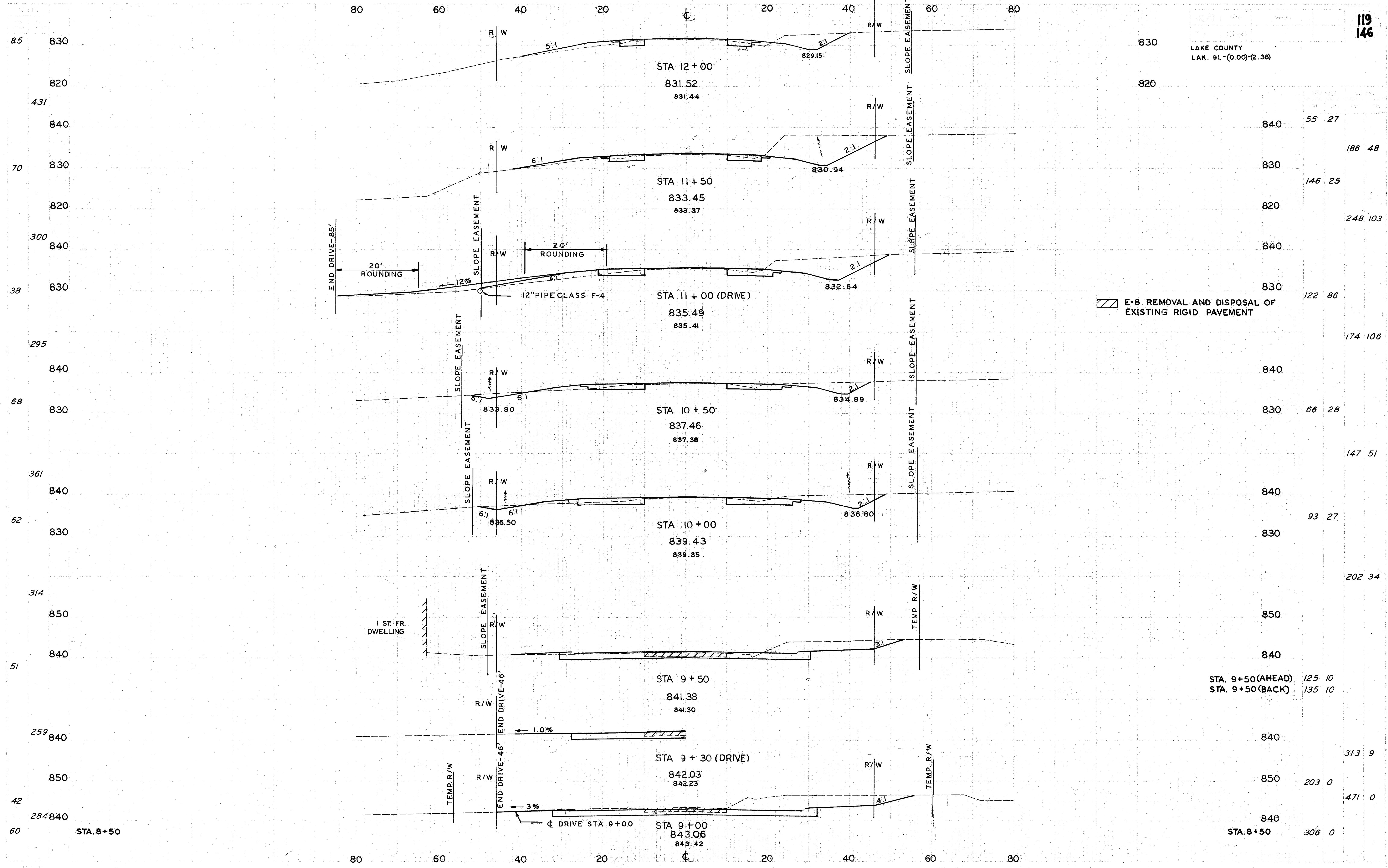
CROSS SECTIONS . . . U.S.R. 6 . . . STA 9+00 TO STA 12+00
