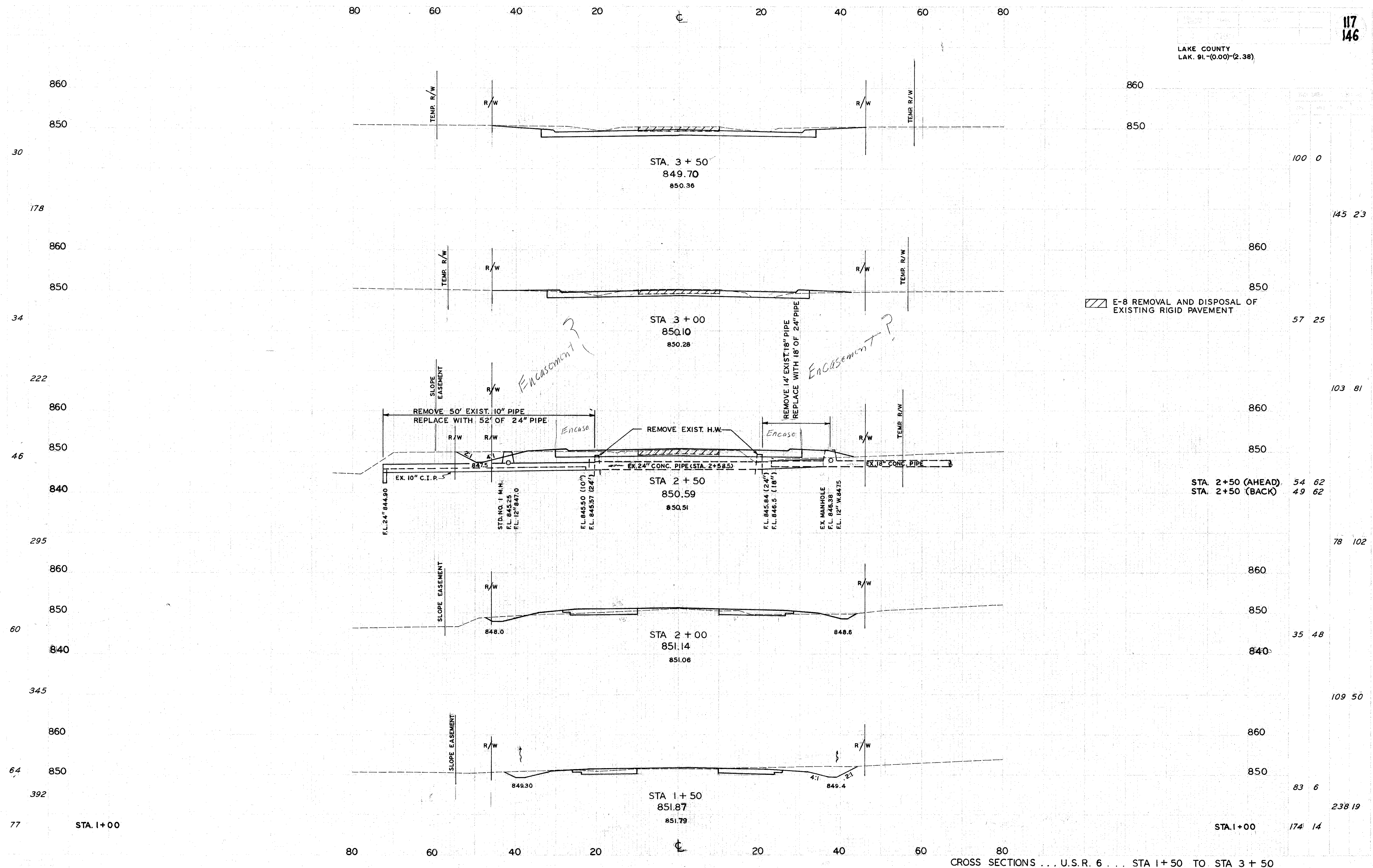
CROSS SECTIONS ... U.S.R. 6 ... STA 1+50 TO STA 3+50
