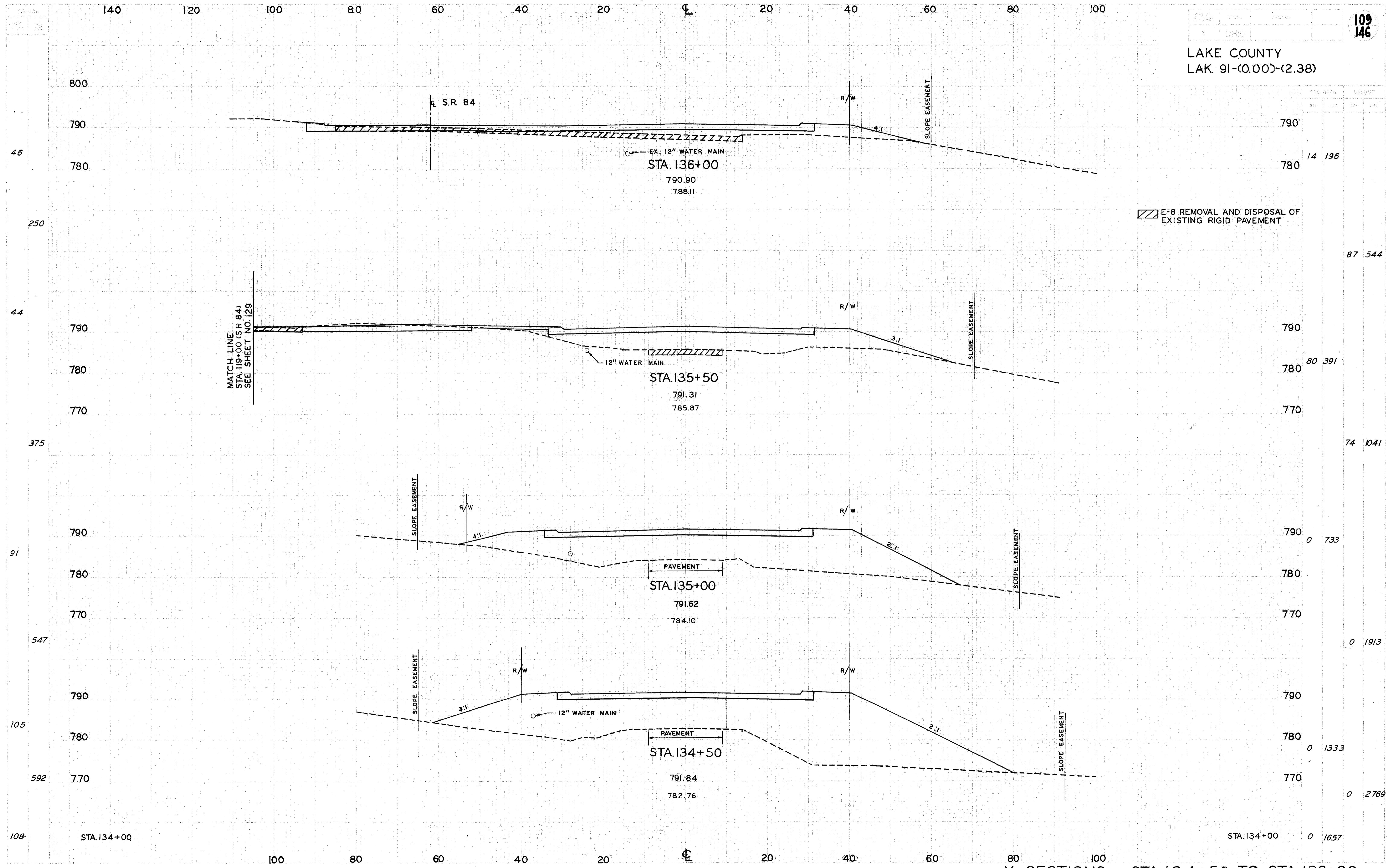
X-SECTIONS STA. 134+50 TO STA. 136+00
