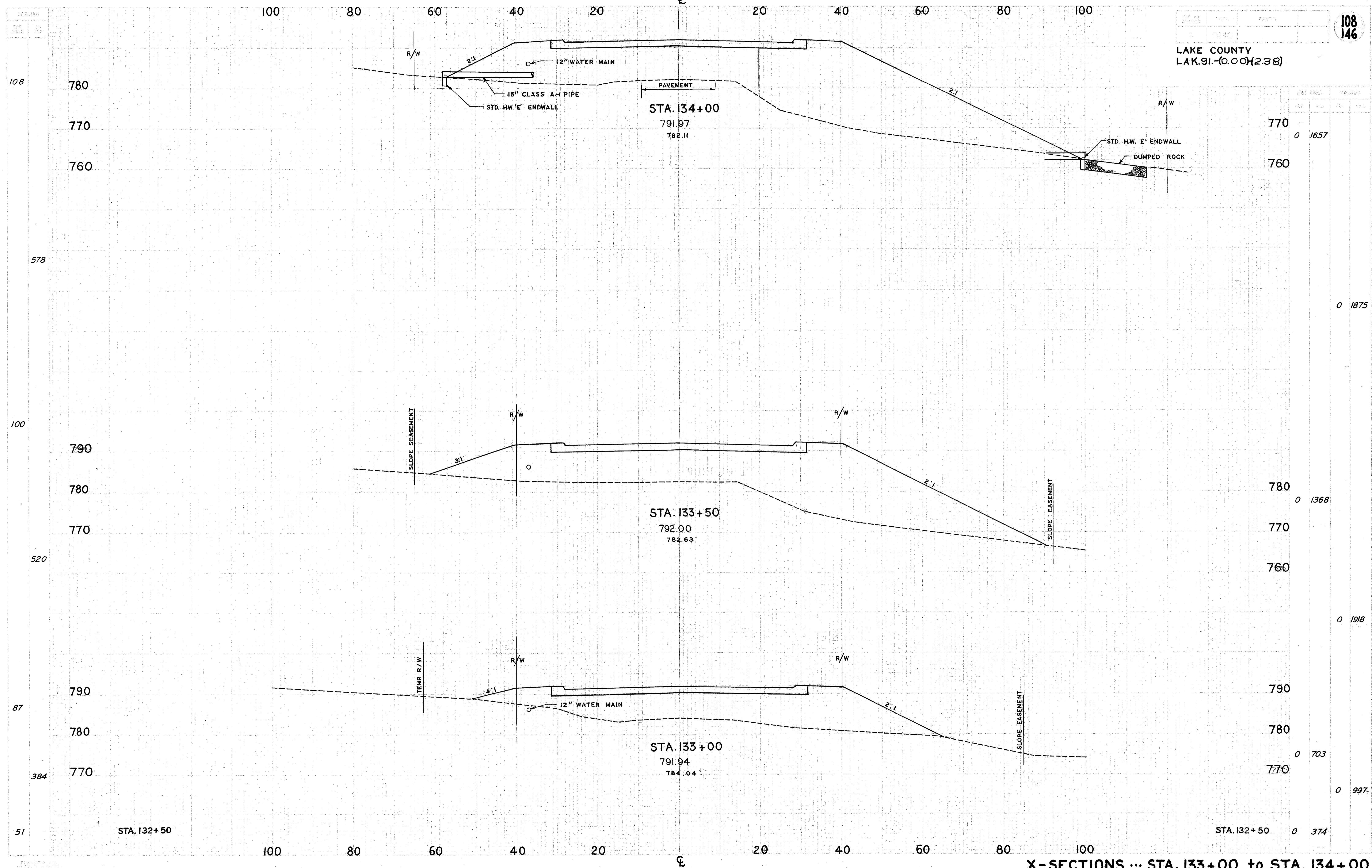
X-SECTIONS ... STA. 133+00 to STA. 134+00
