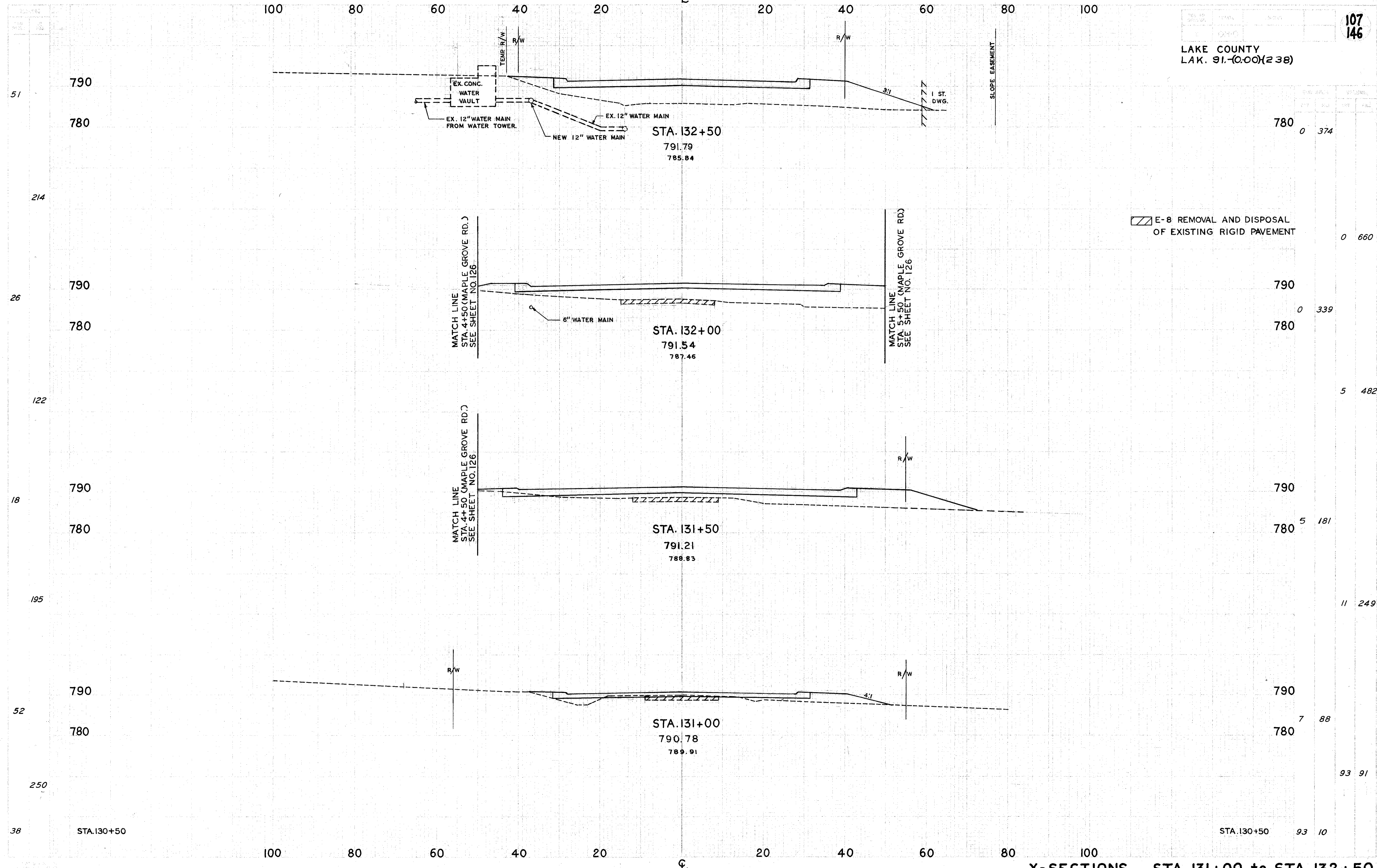
X-SECTIONS ... STA. 131+00 to STA. 132+50
