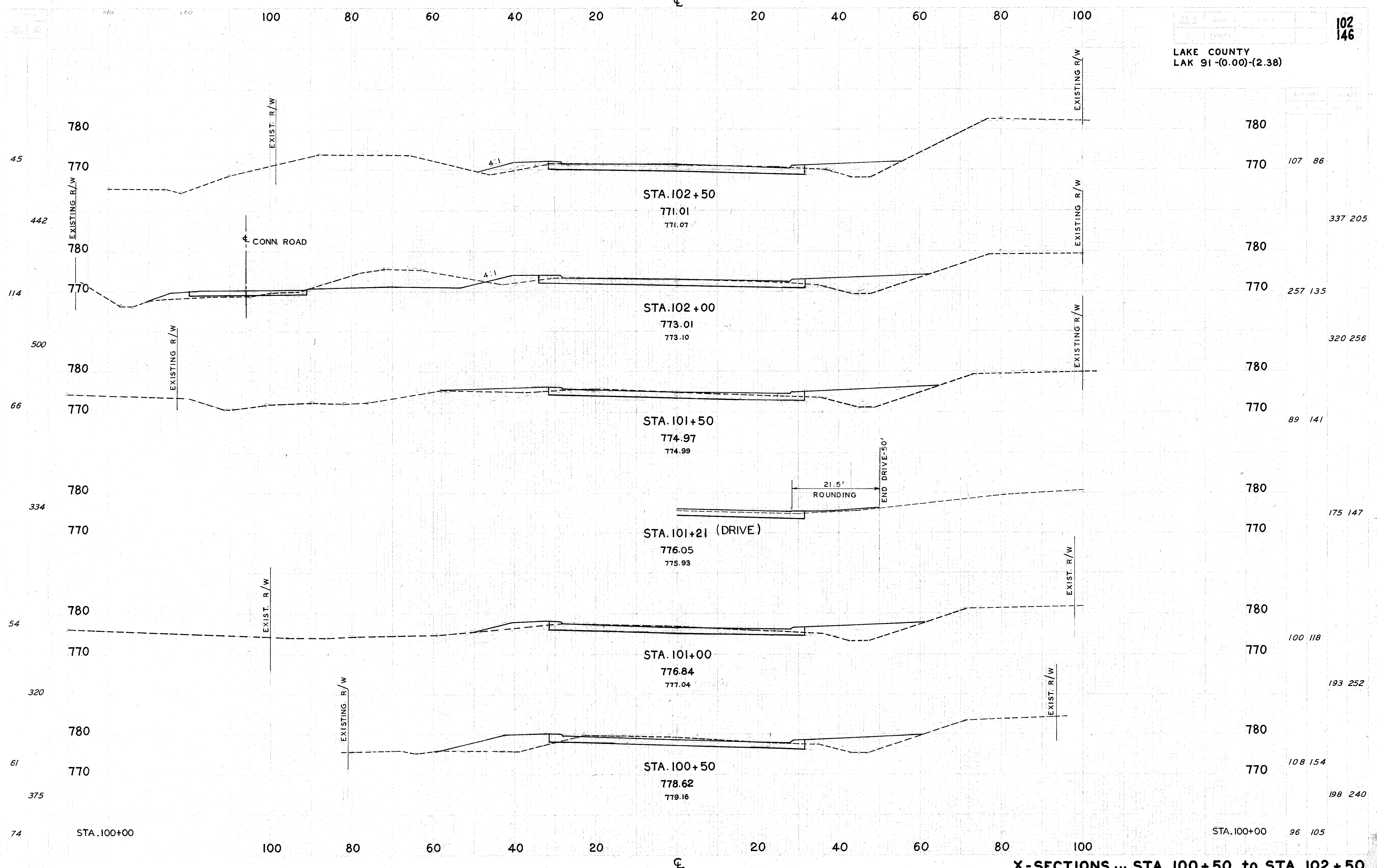
X-SECTIONS ... STA. 100+50 to STA. 102+50
