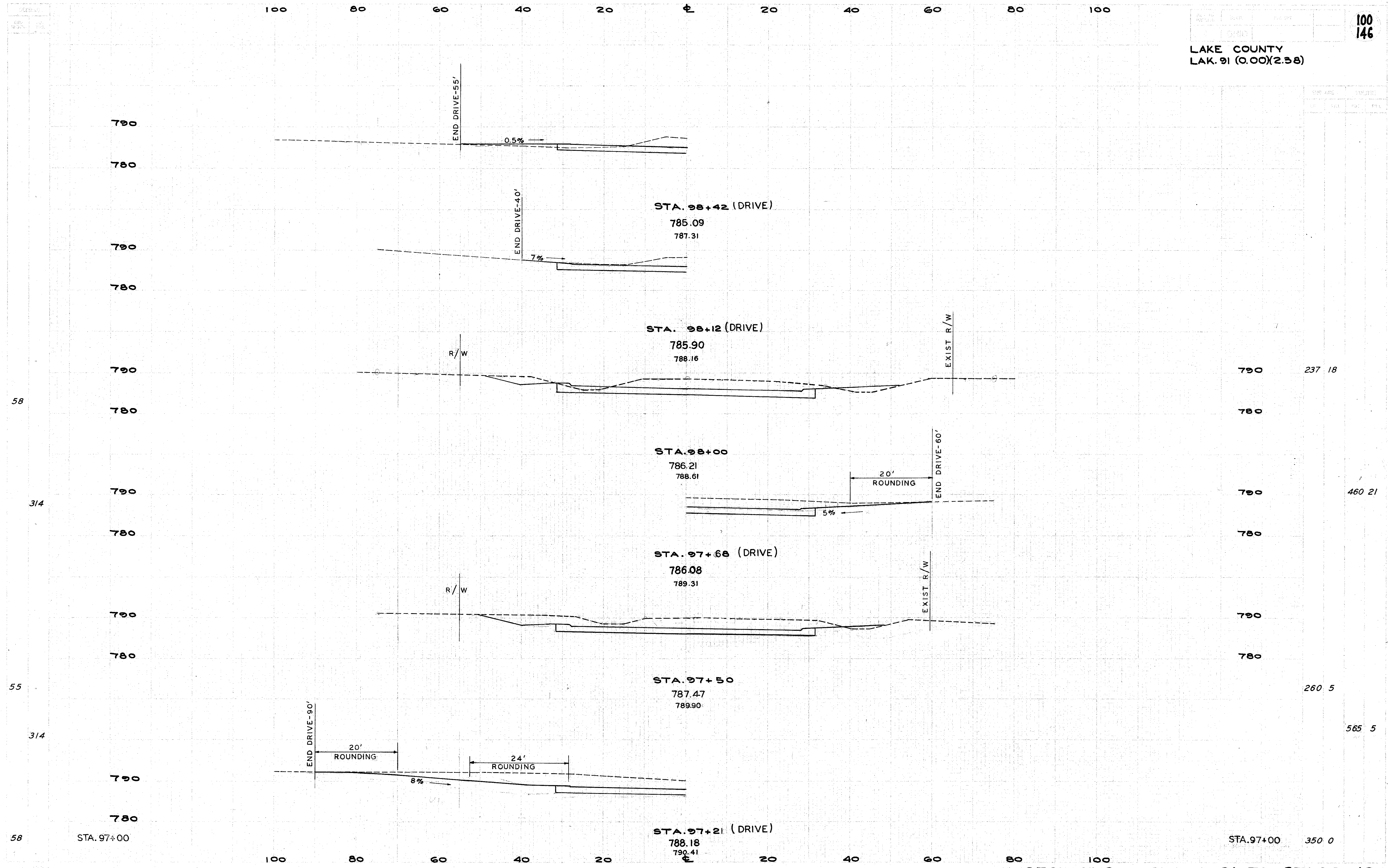
X-SECTIONS STA. 97+21 TO STA. 98+42
