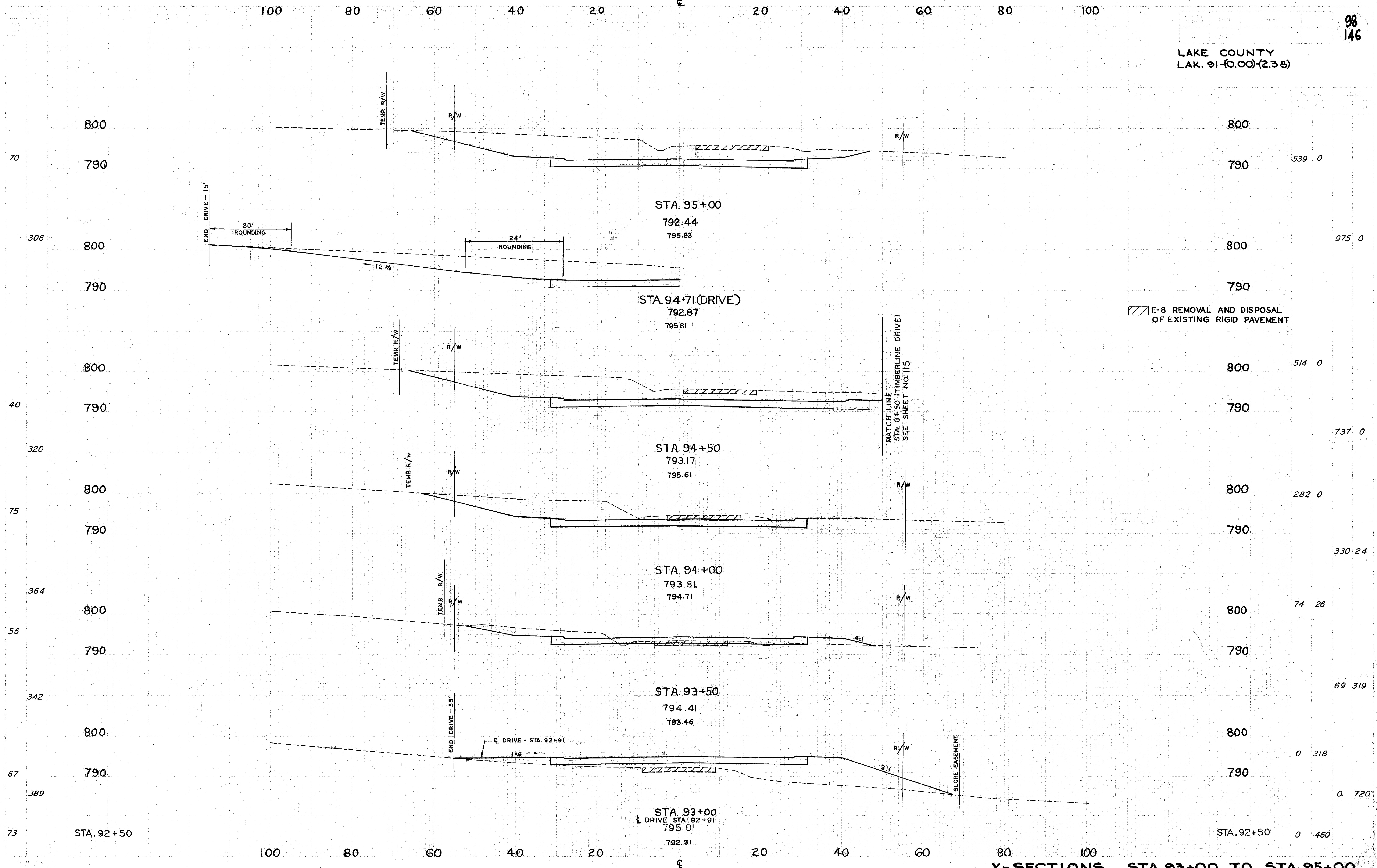
X-SECTIONS STA. 93+00 TO STA. 95+00
