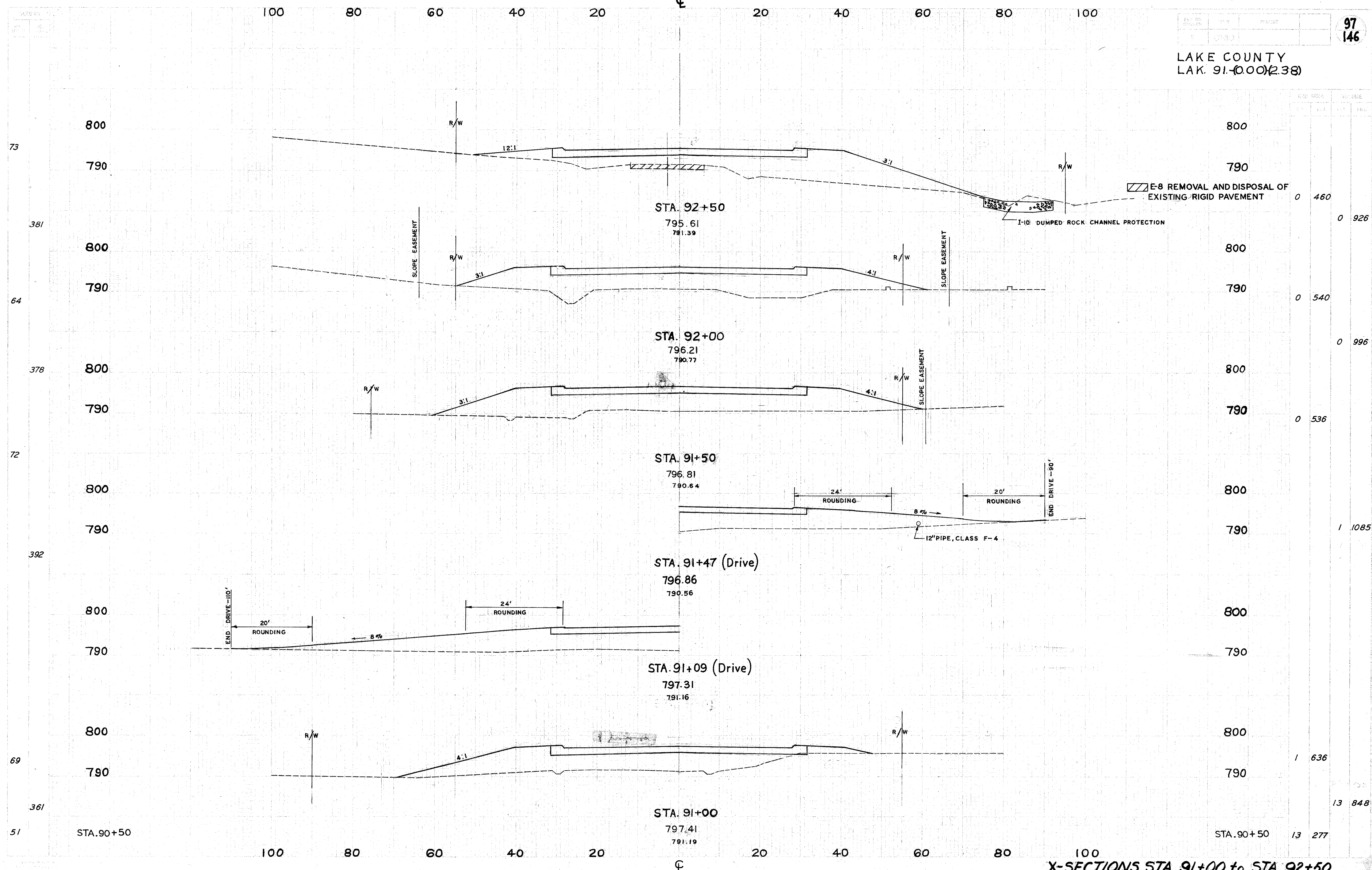
X-SECTIONS STA. 91+00 to STA. 92+50
