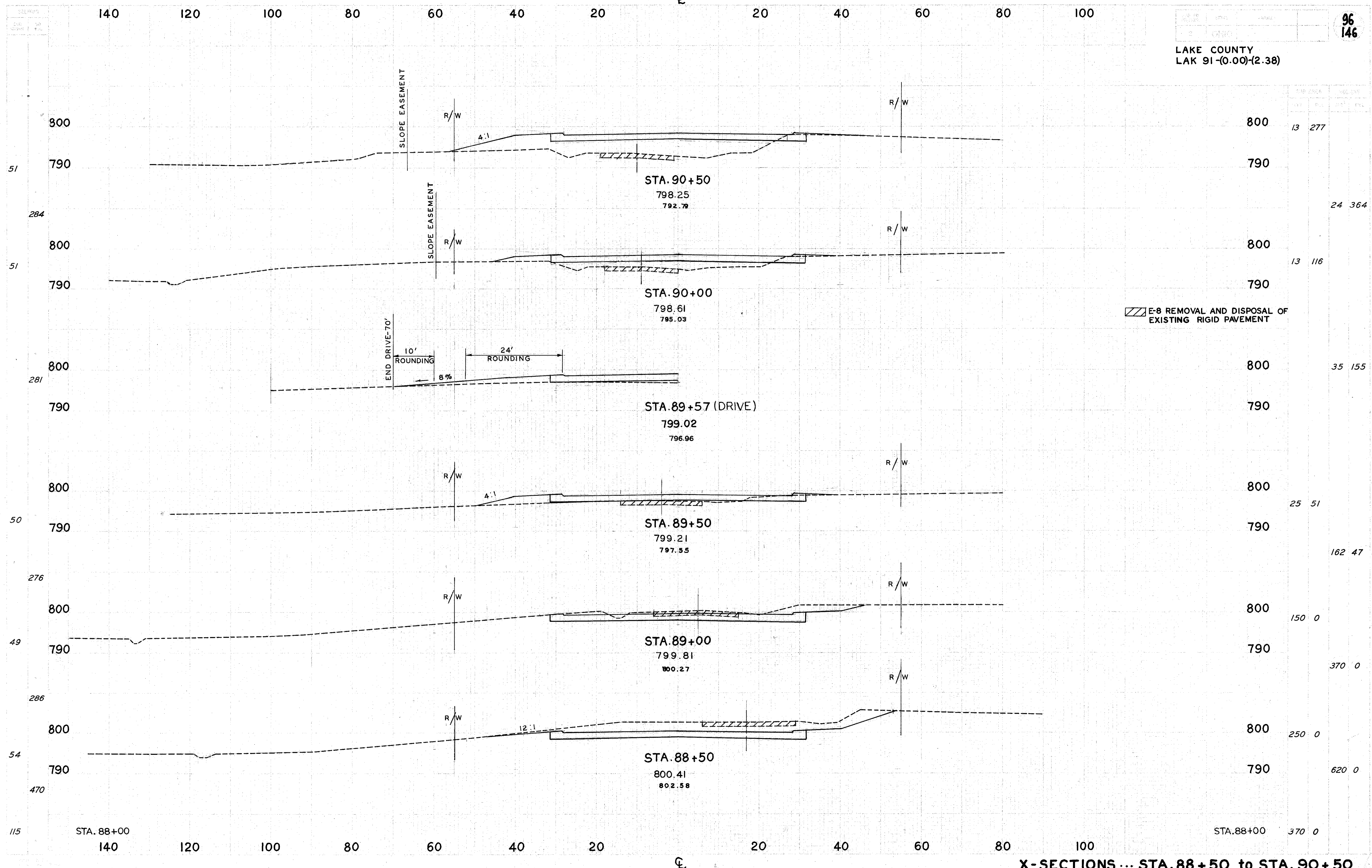
X-SECTIONS ... STA. 88+50 to STA. 90+50
