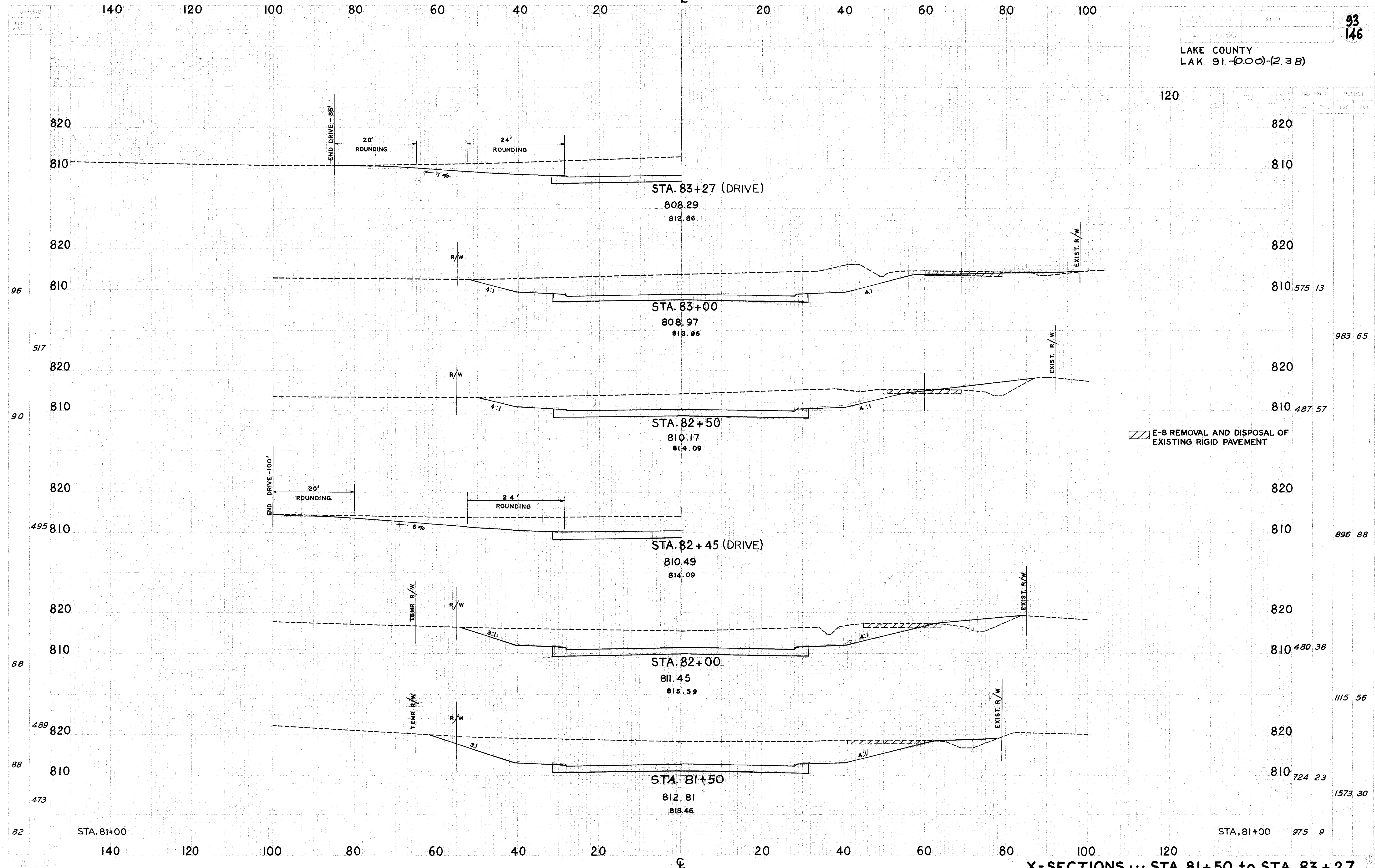
X-SECTIONS ... STA. 81+50 to STA. 83+27
