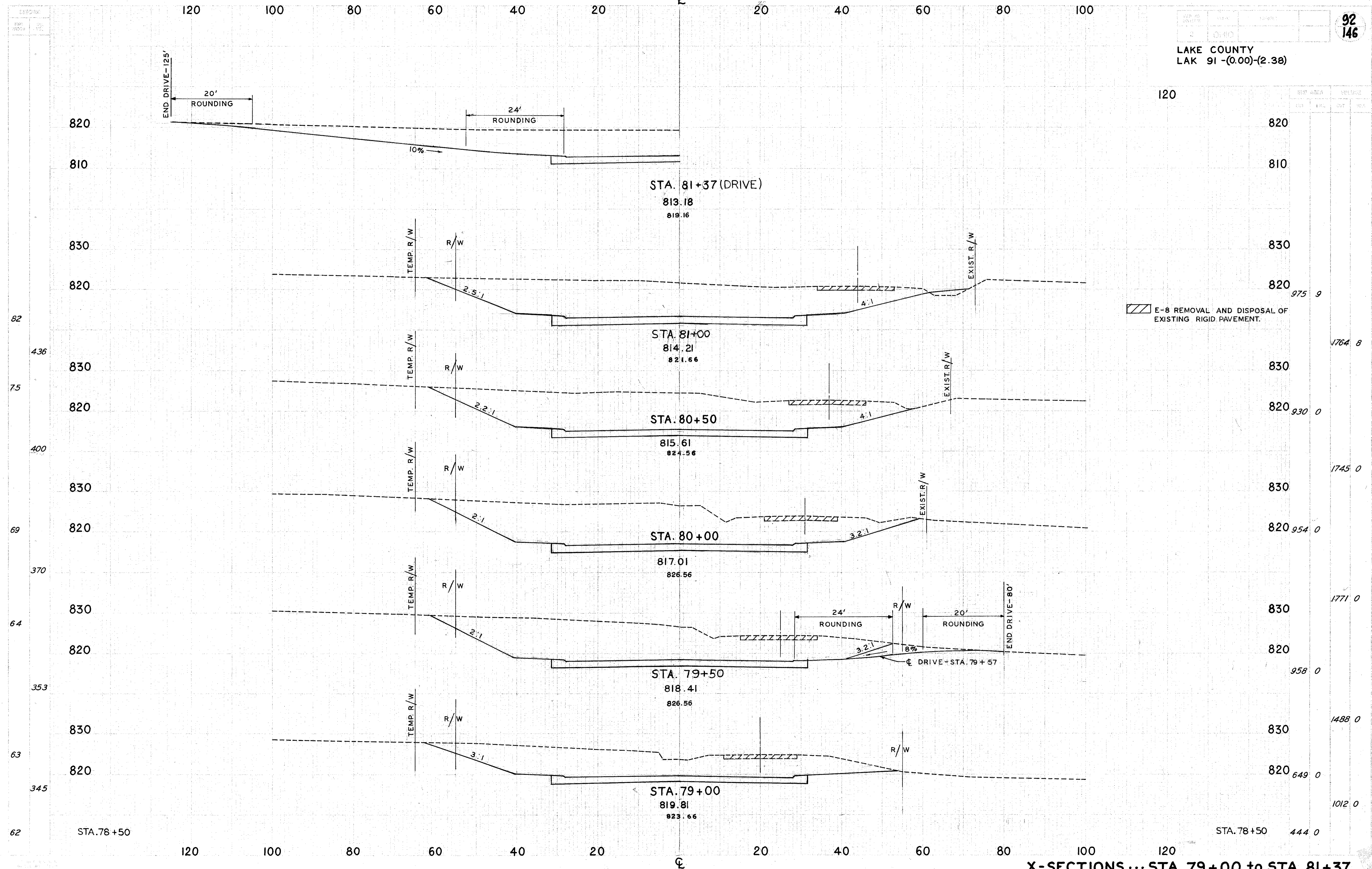
X-SECTIONS ... STA. 79+00 to STA. 81+37
