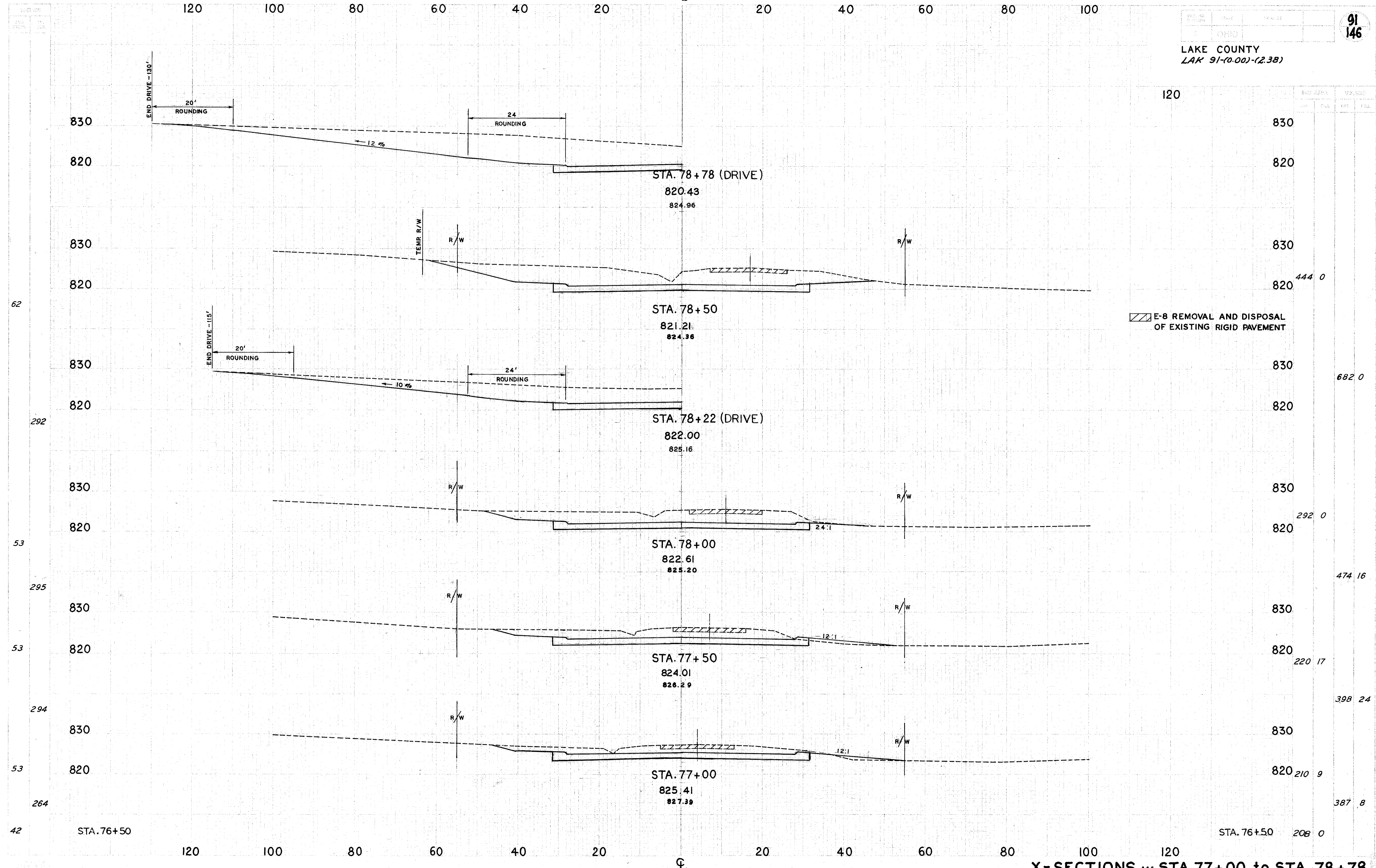
X-SECTIONS ... STA. 77+00 to STA. 78+78
