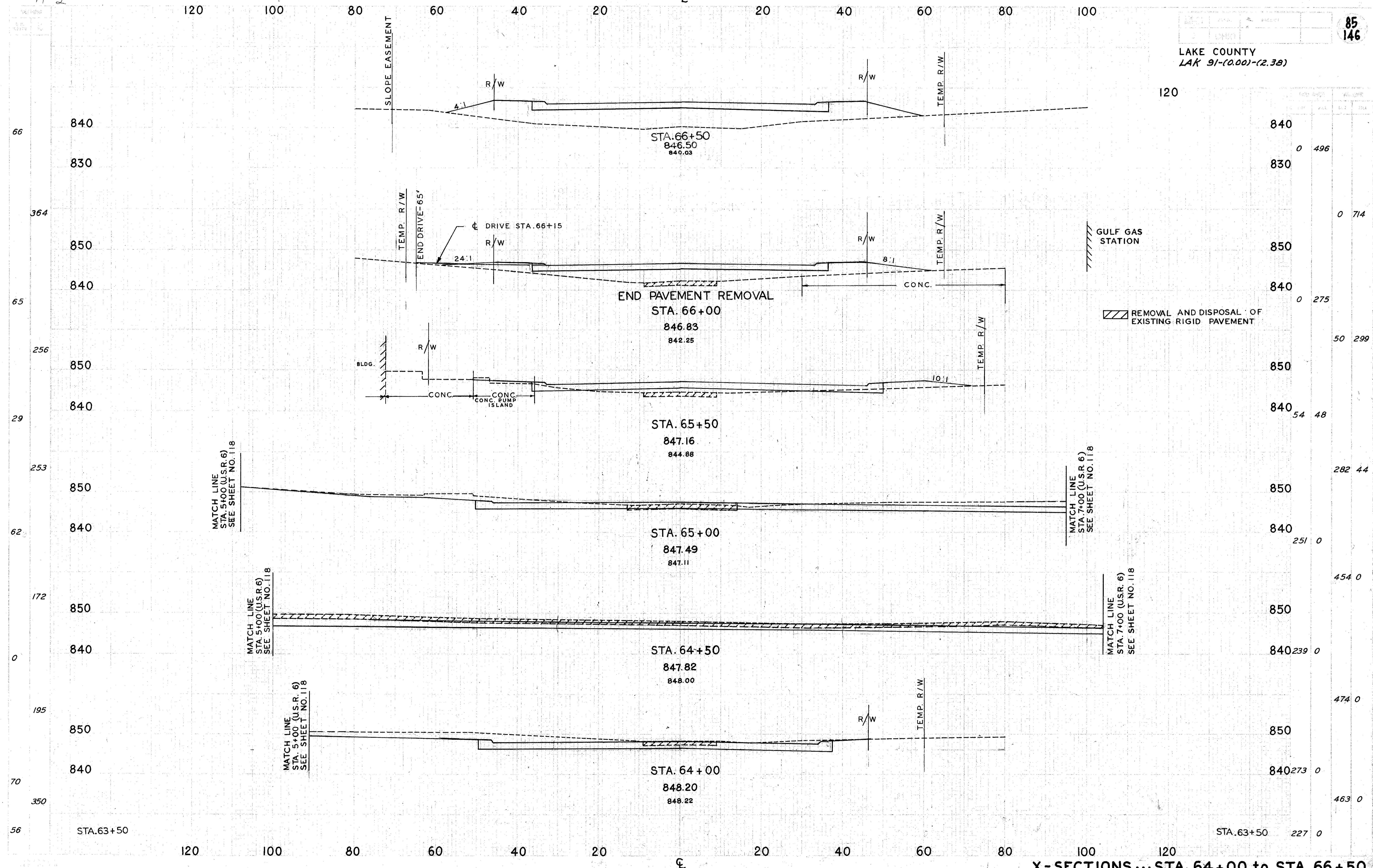
X-SECTIONS ... STA. 64+00 to STA. 66+50
