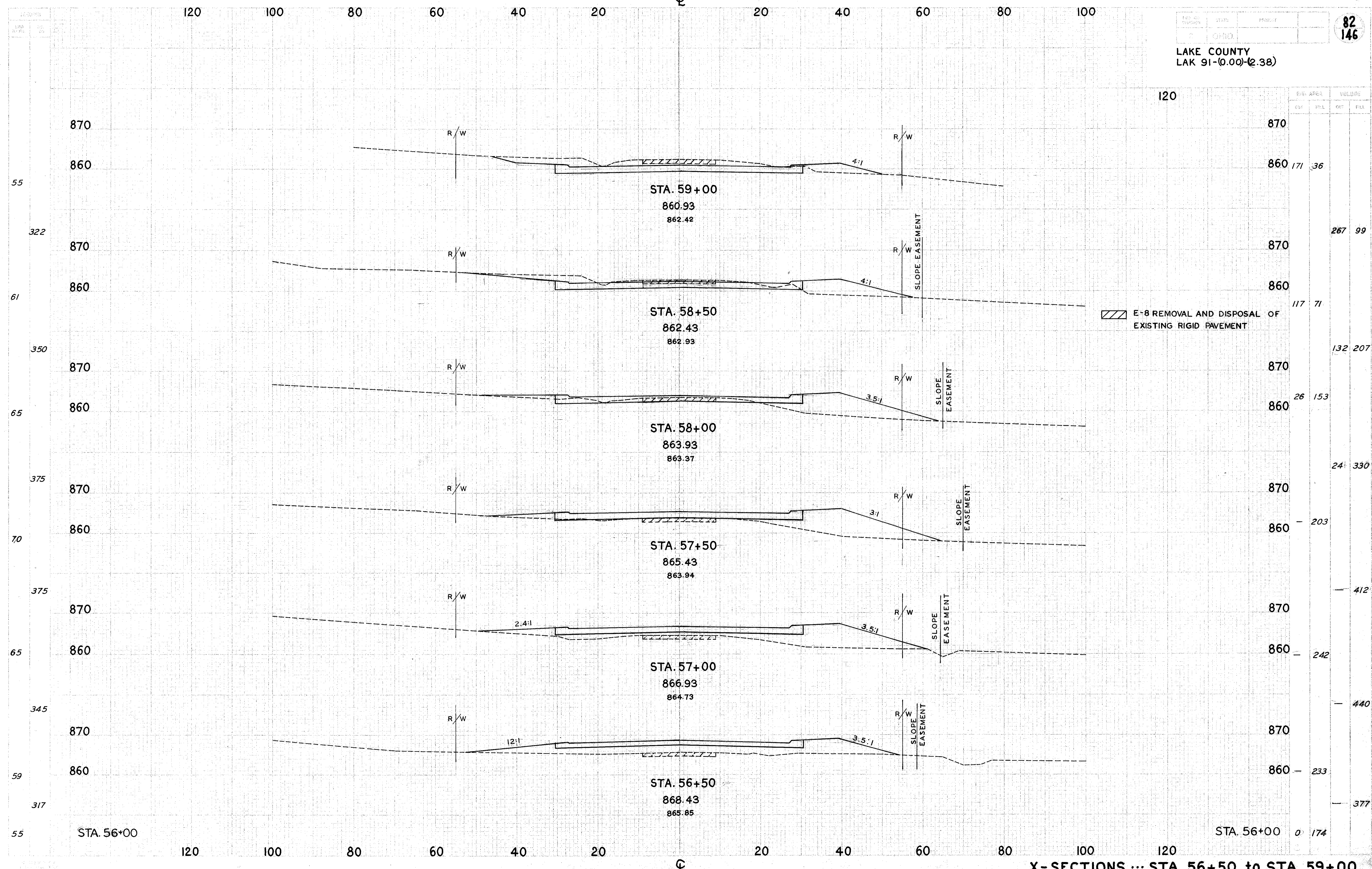
X-SECTIONS ... STA. 56+50 to STA. 59+00
