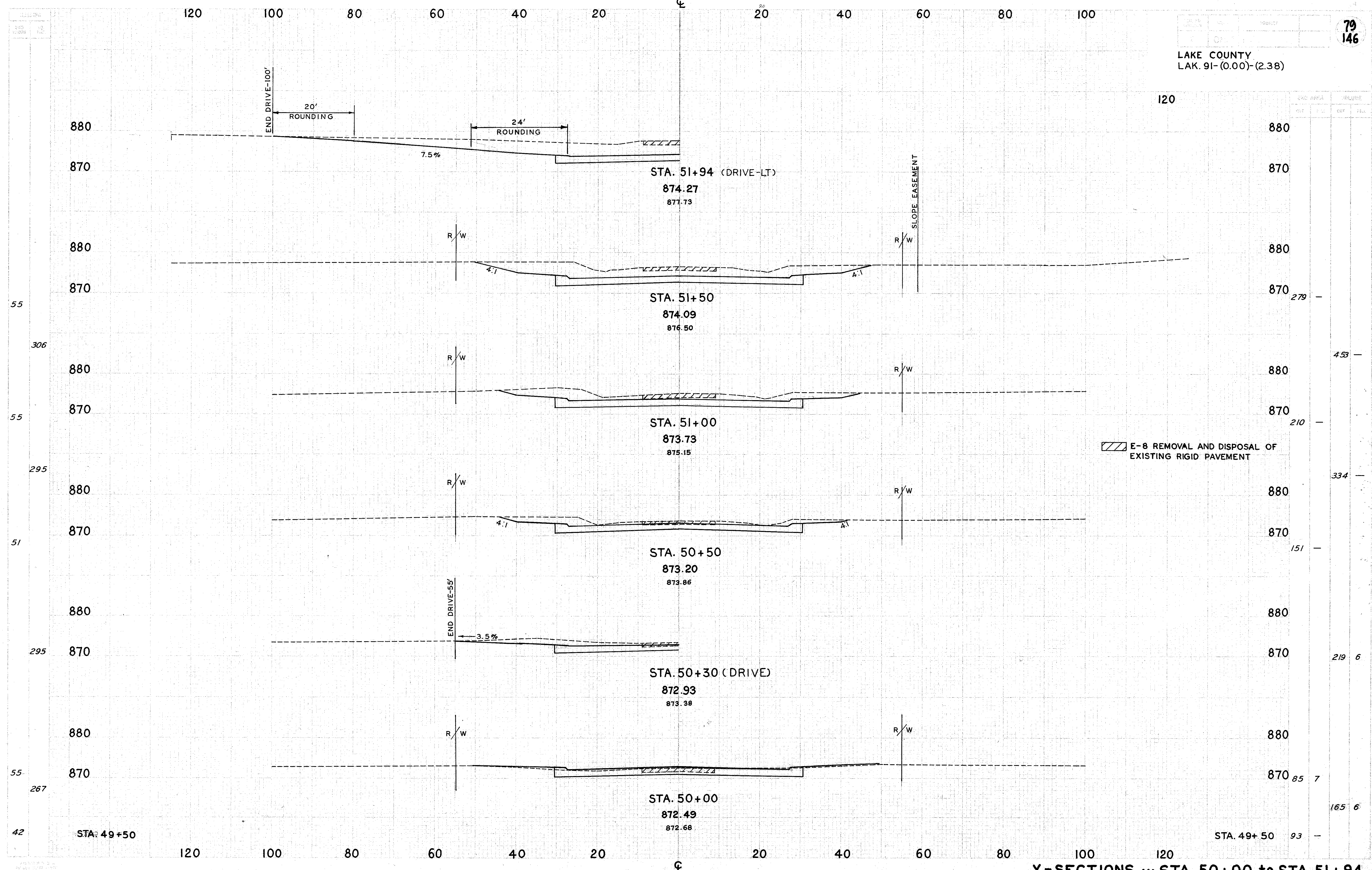
X-SECTIONS ... STA. 50+00 to STA. 51+94
