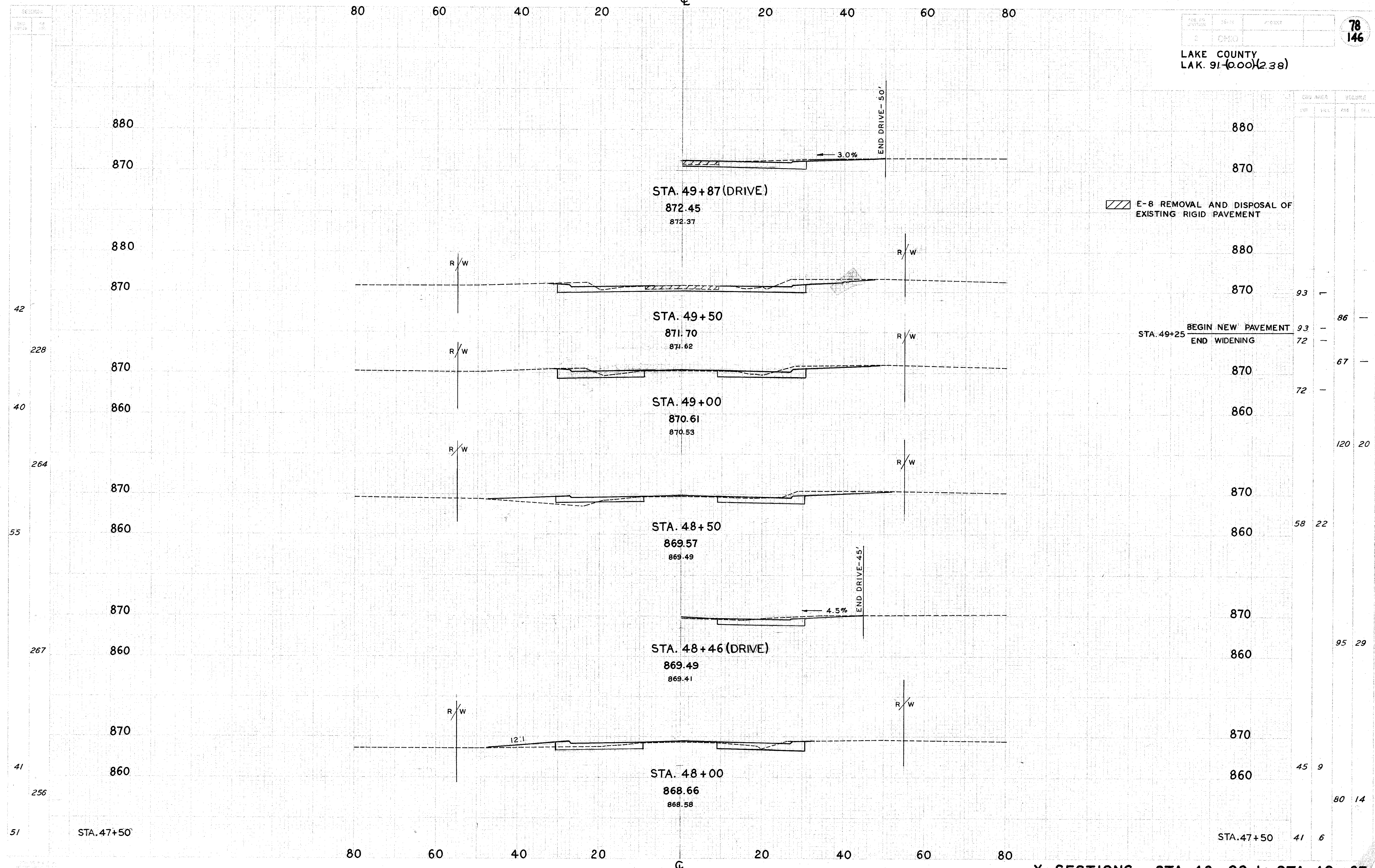
X-SECTIONS ... STA. 48+00 to STA. 49+87
