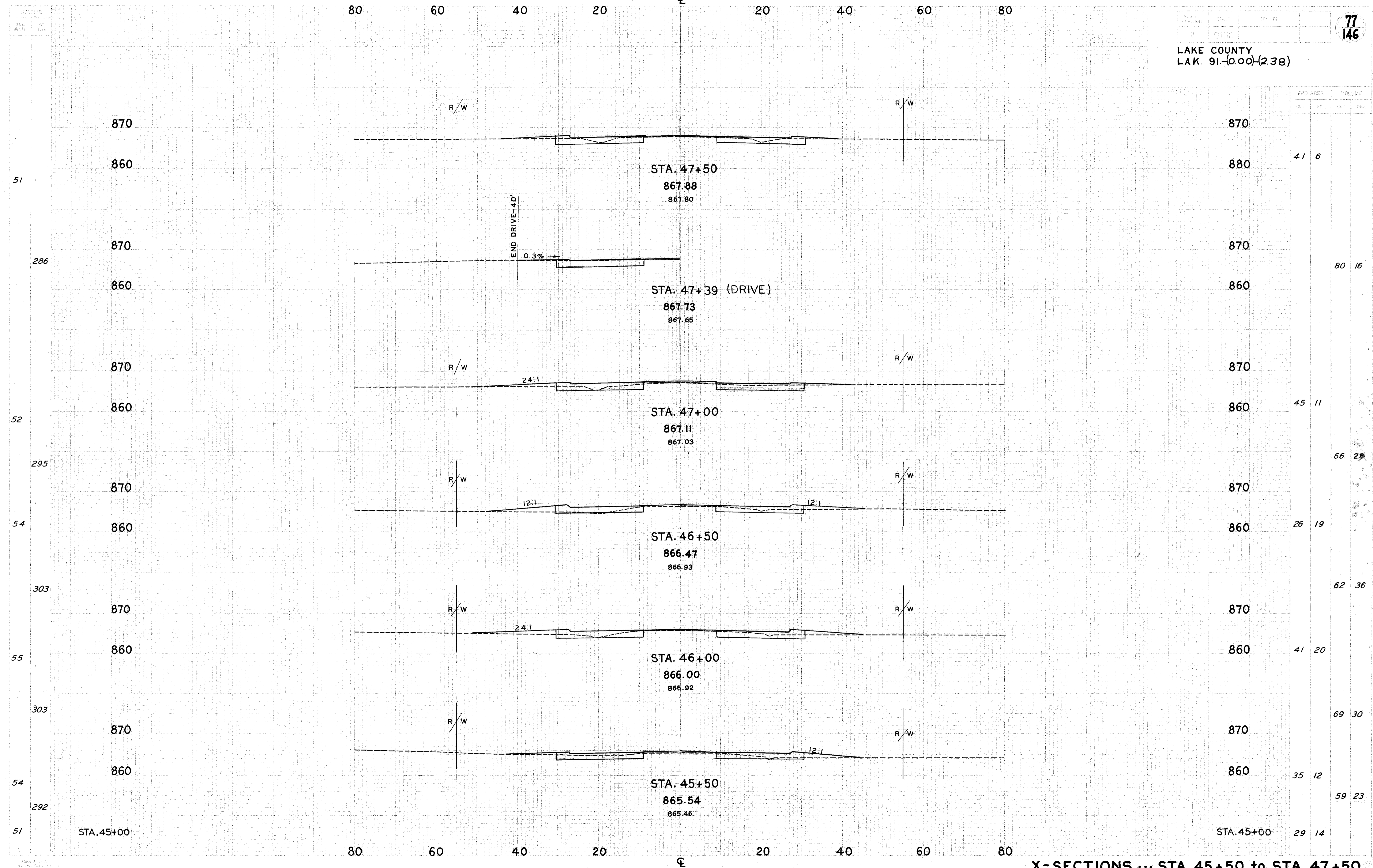
X-SECTIONS ... STA. 45+50 to STA. 47+50
