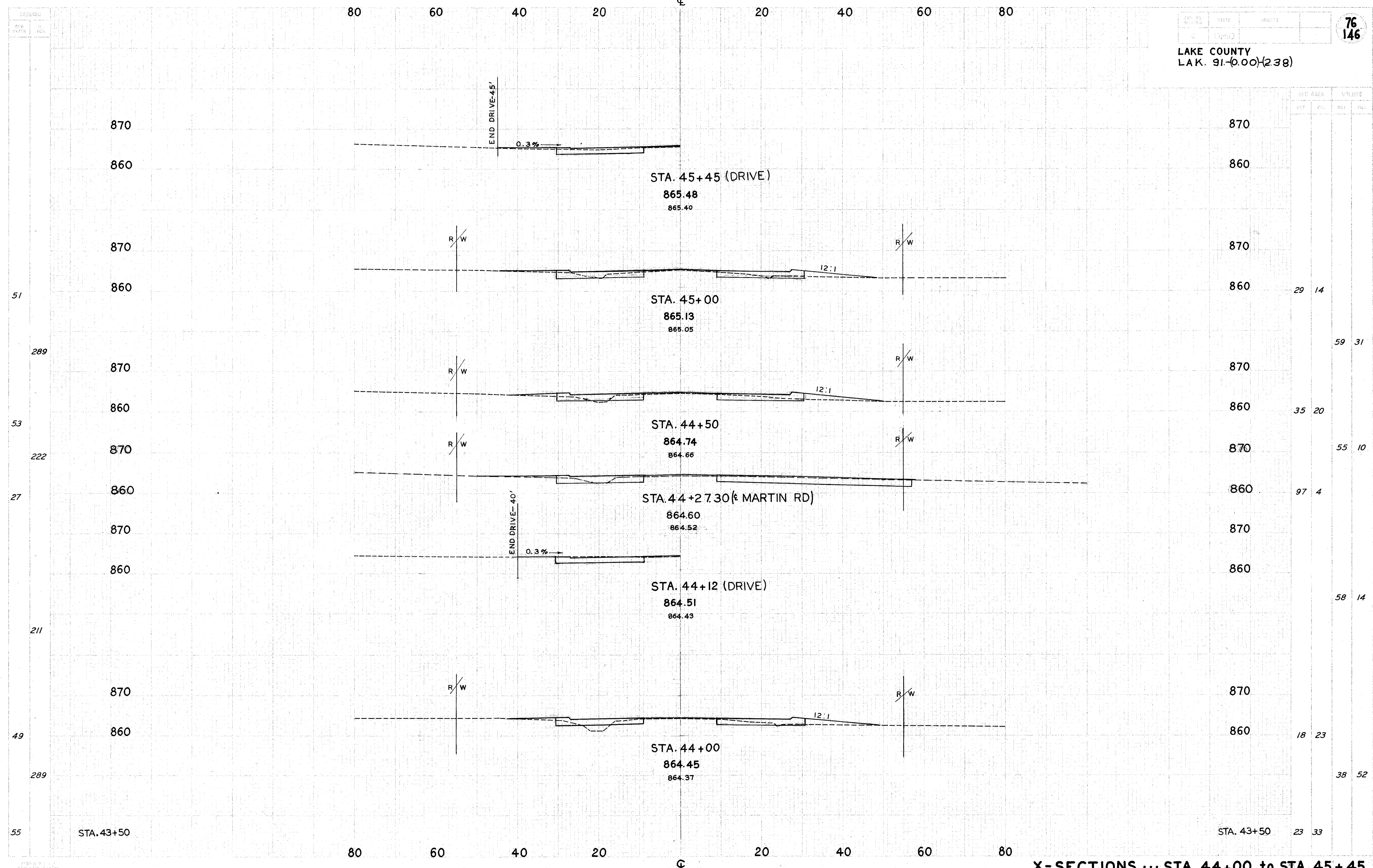
X-SECTIONS ... STA. 44+00 to STA. 45+45
