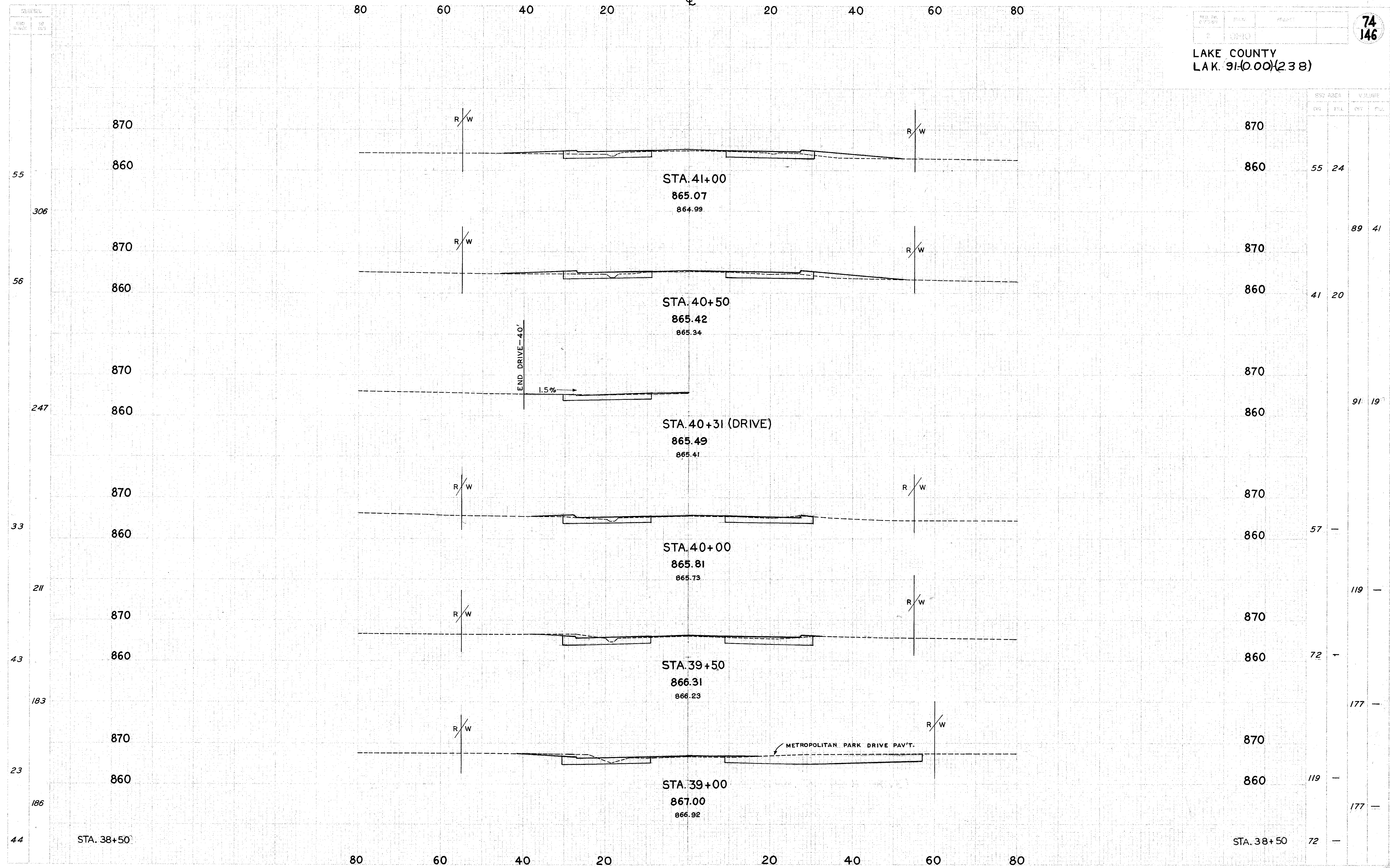
X-SECTIONS STA. 39+00 to STA. 41+00
