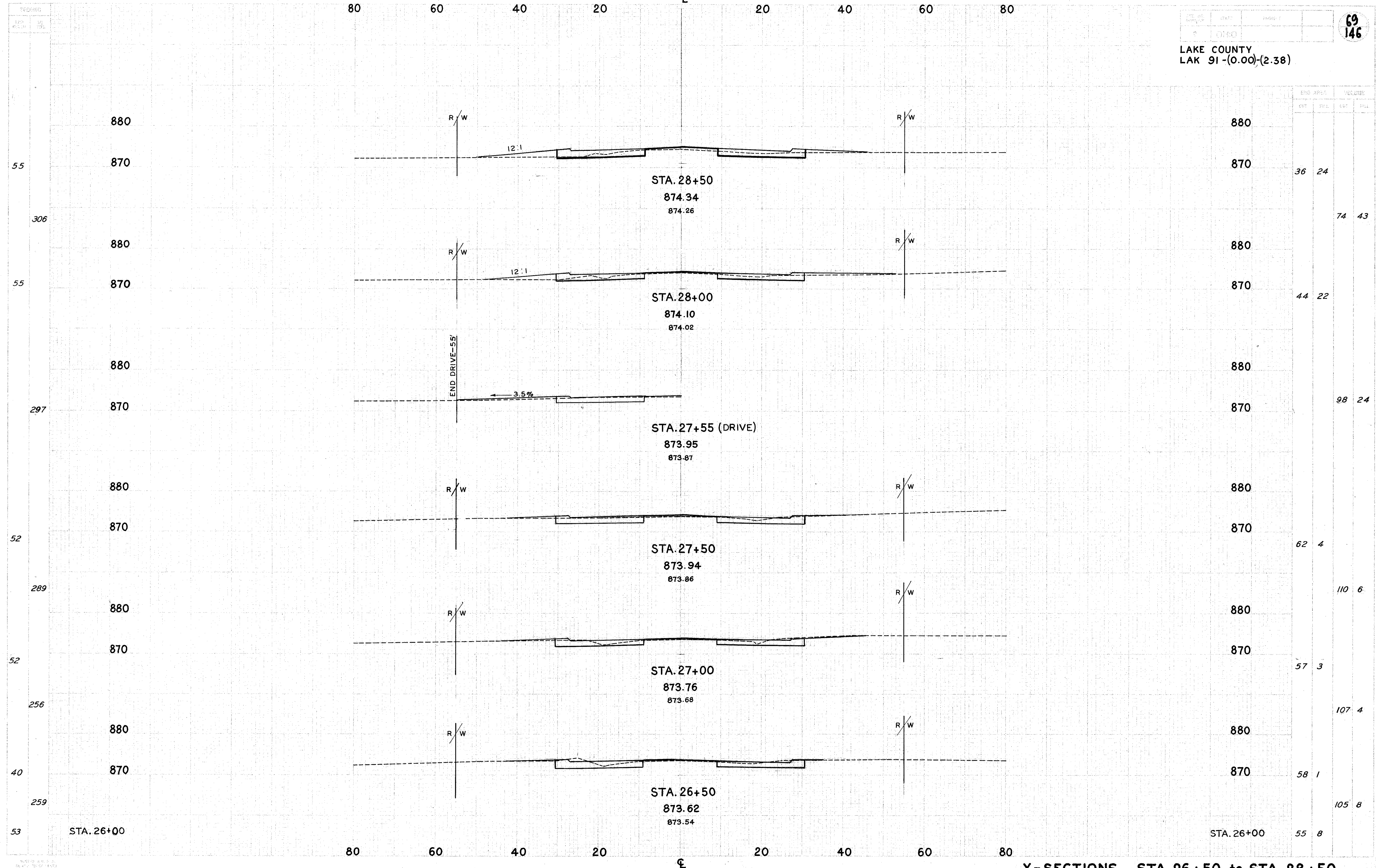
X-SECTIONS ... STA. 26+50 to STA. 28+50
