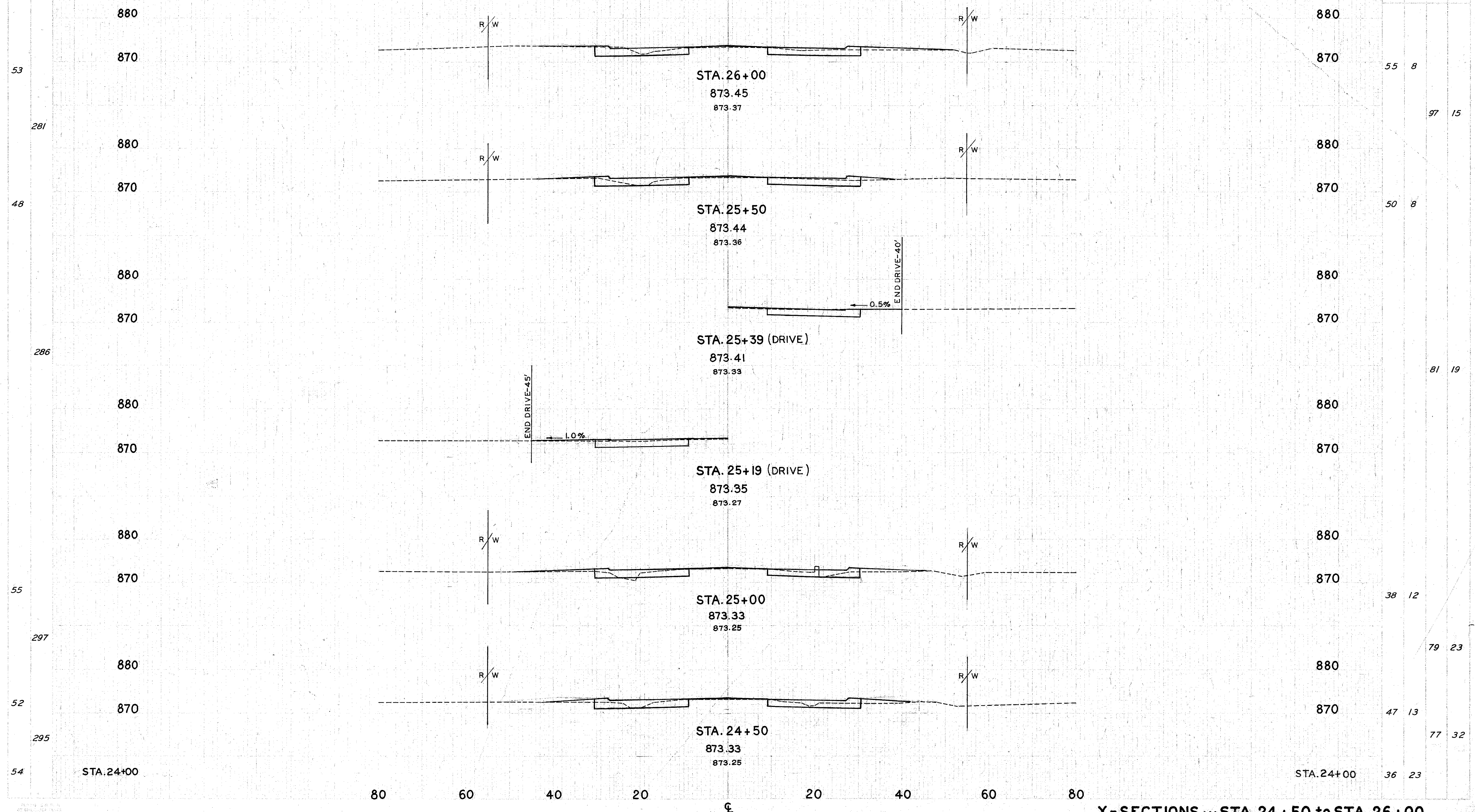
X-SECTIONS ... STA. 24+50 to STA. 26+00
