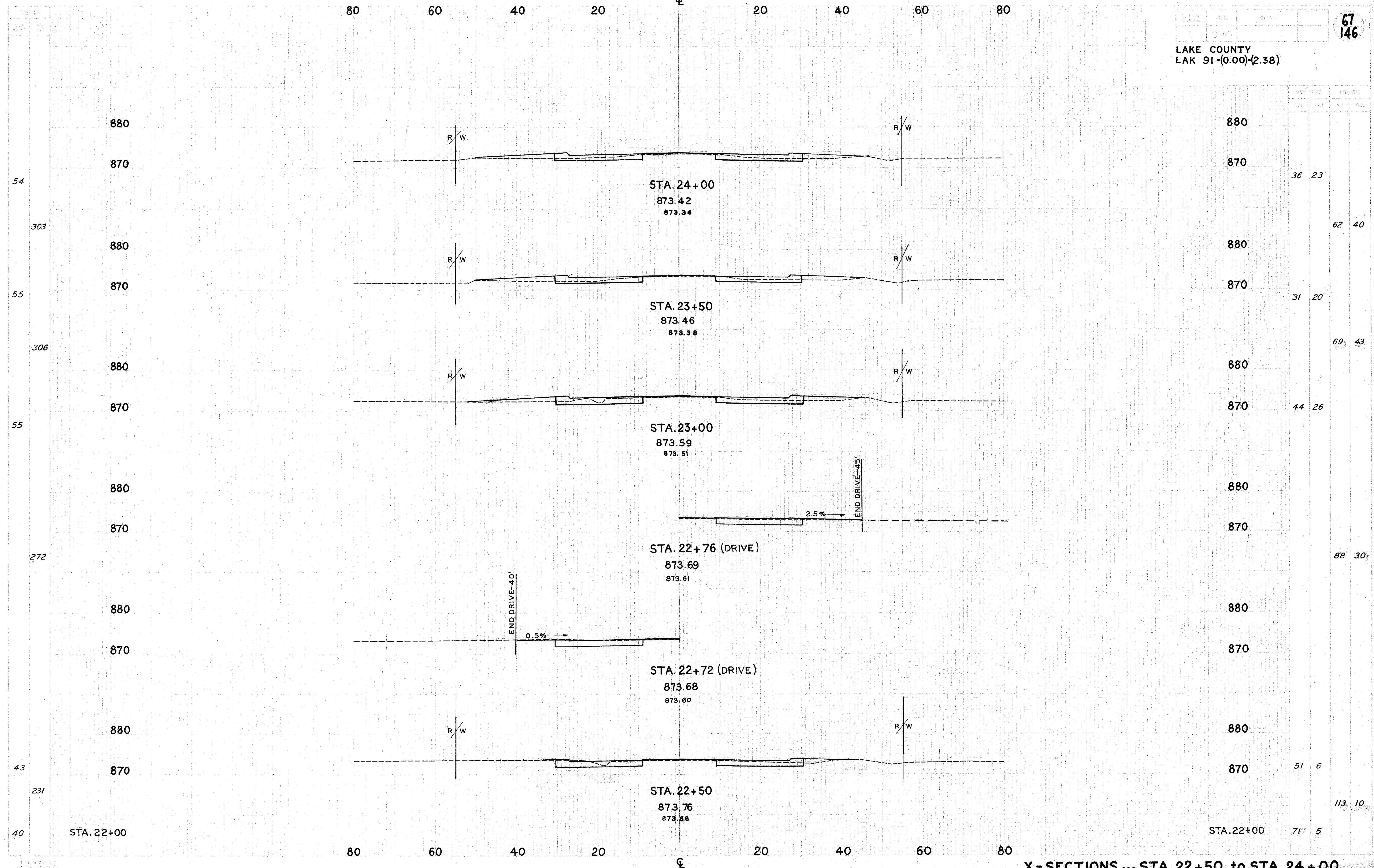
X-SECTIONS ... STA. 22+50 to STA. 24+00
