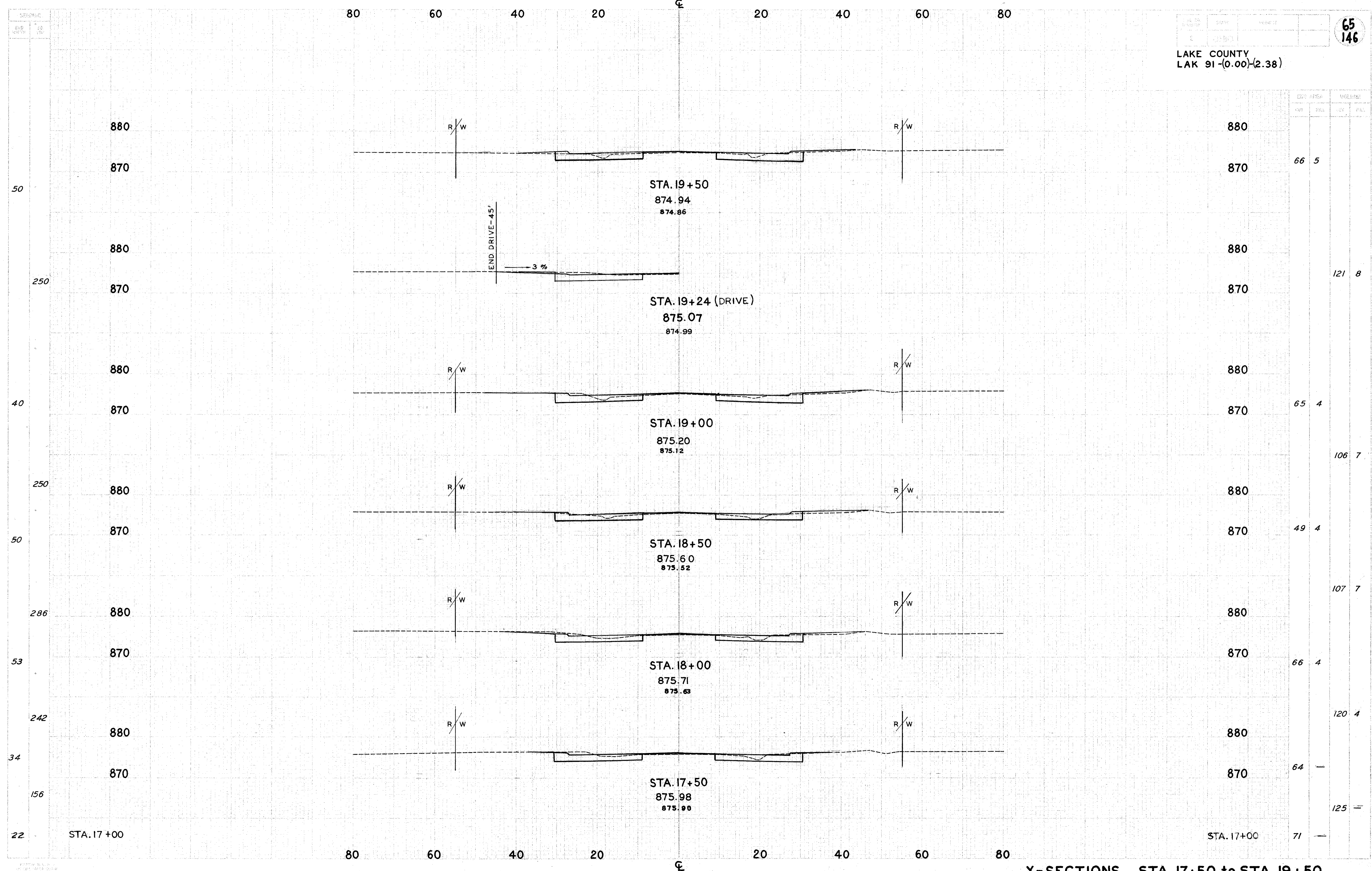
X-SECTIONS ... STA. 17+50 to STA. 19+50
