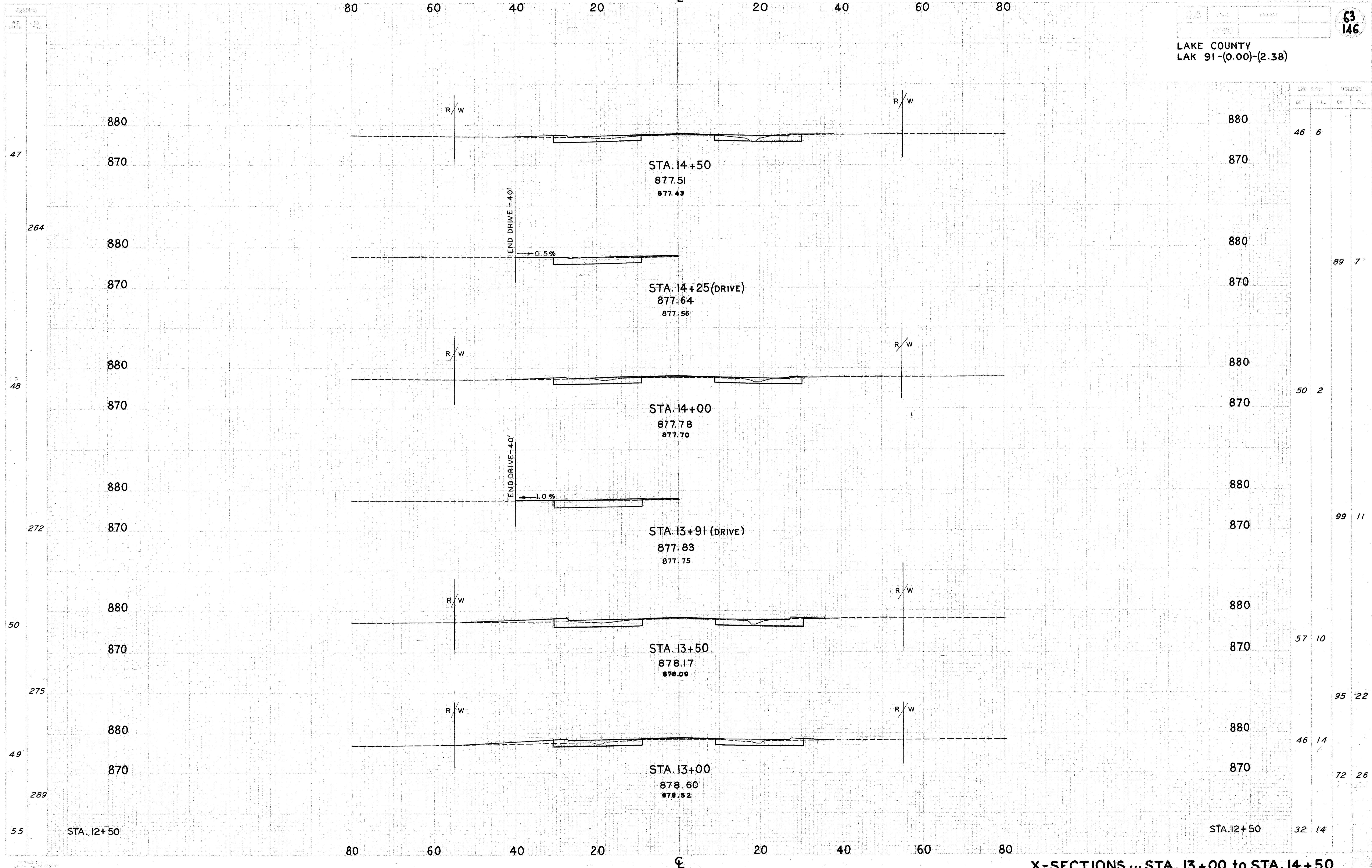
X-SECTIONS ... STA. 13+00 to STA. 14+50
