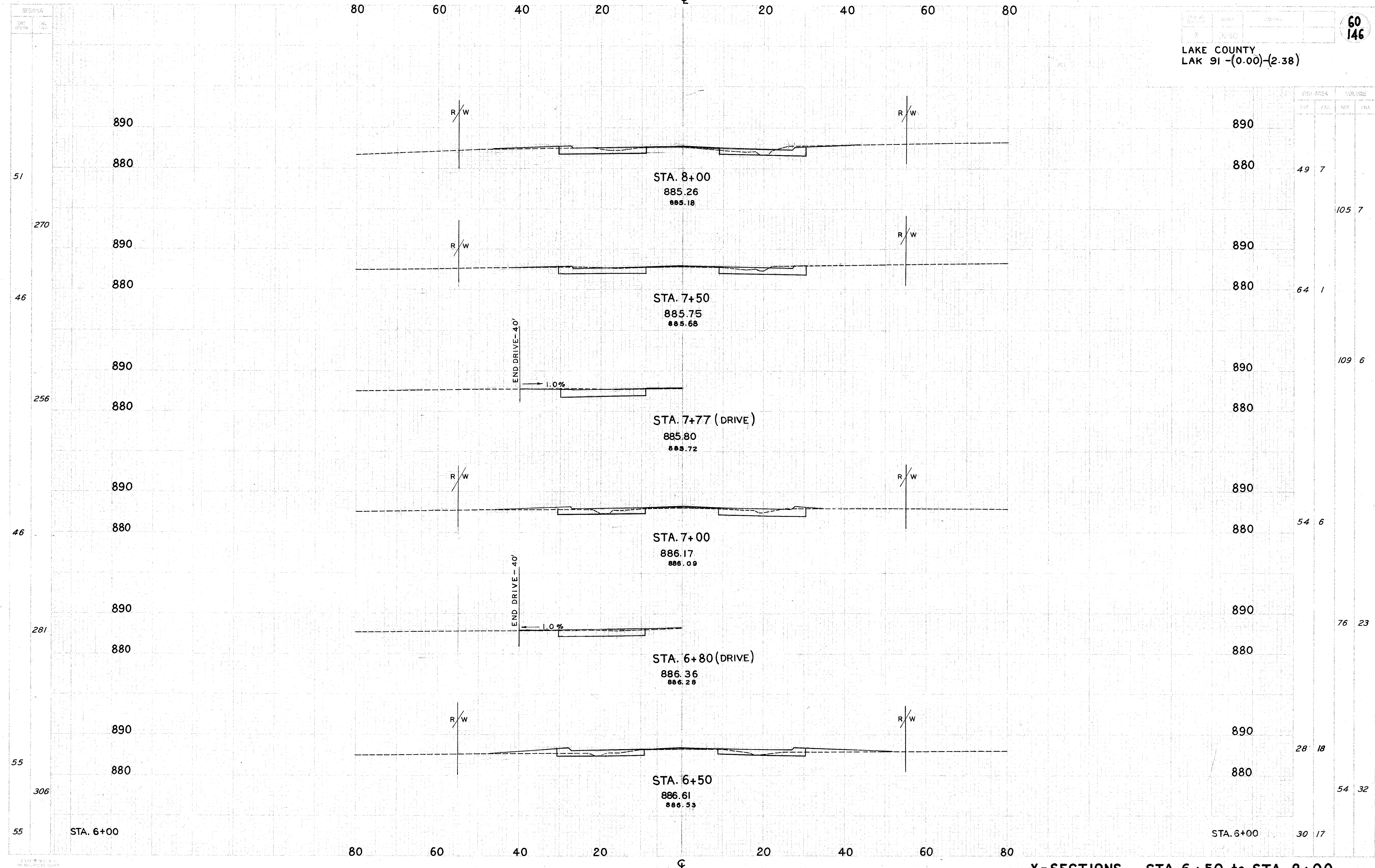
X-SECTIONS ... STA. 6+50 to STA. 8+00
