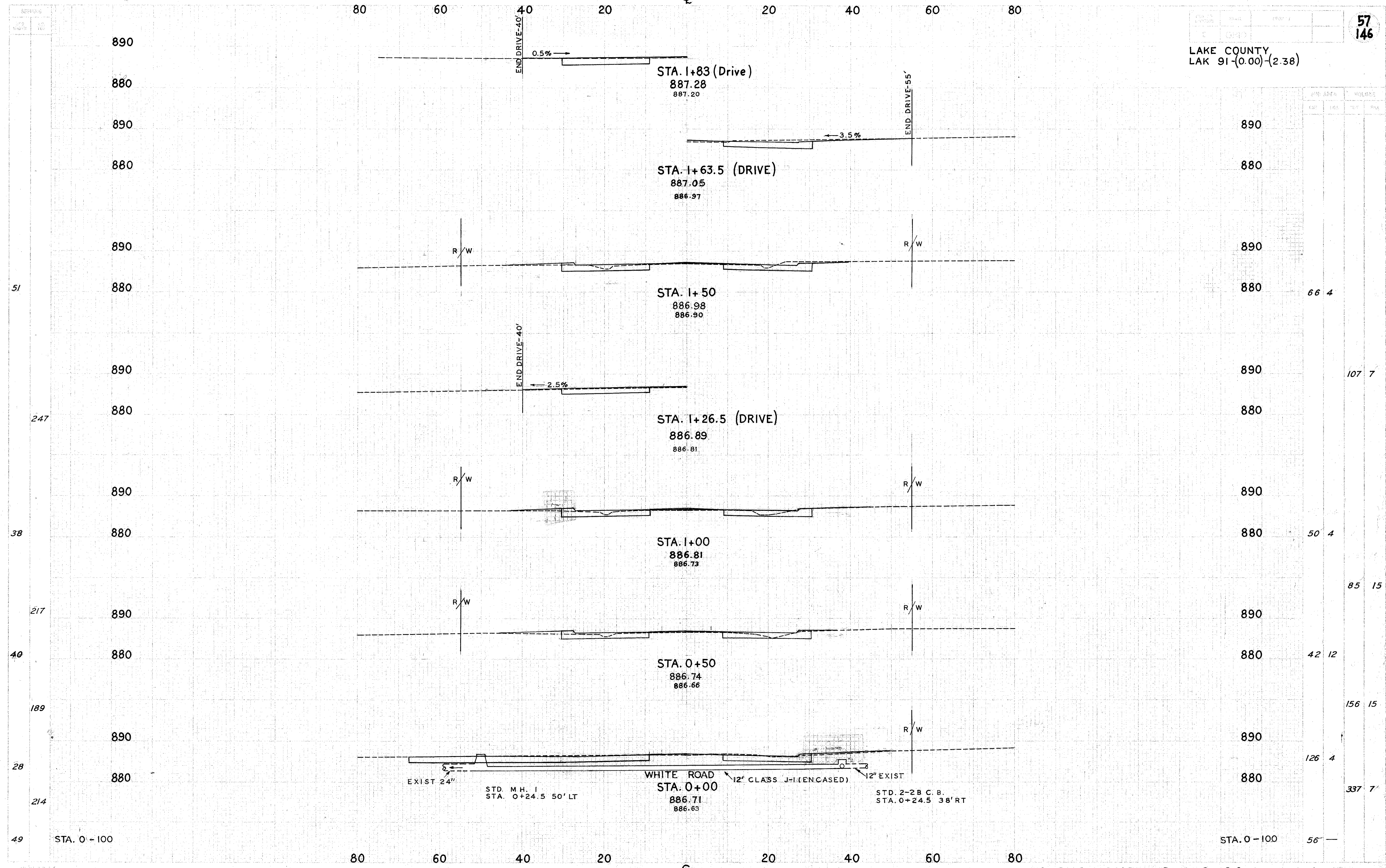
X-SECTIONS ... STA. 0+00 to STA. 1+83
