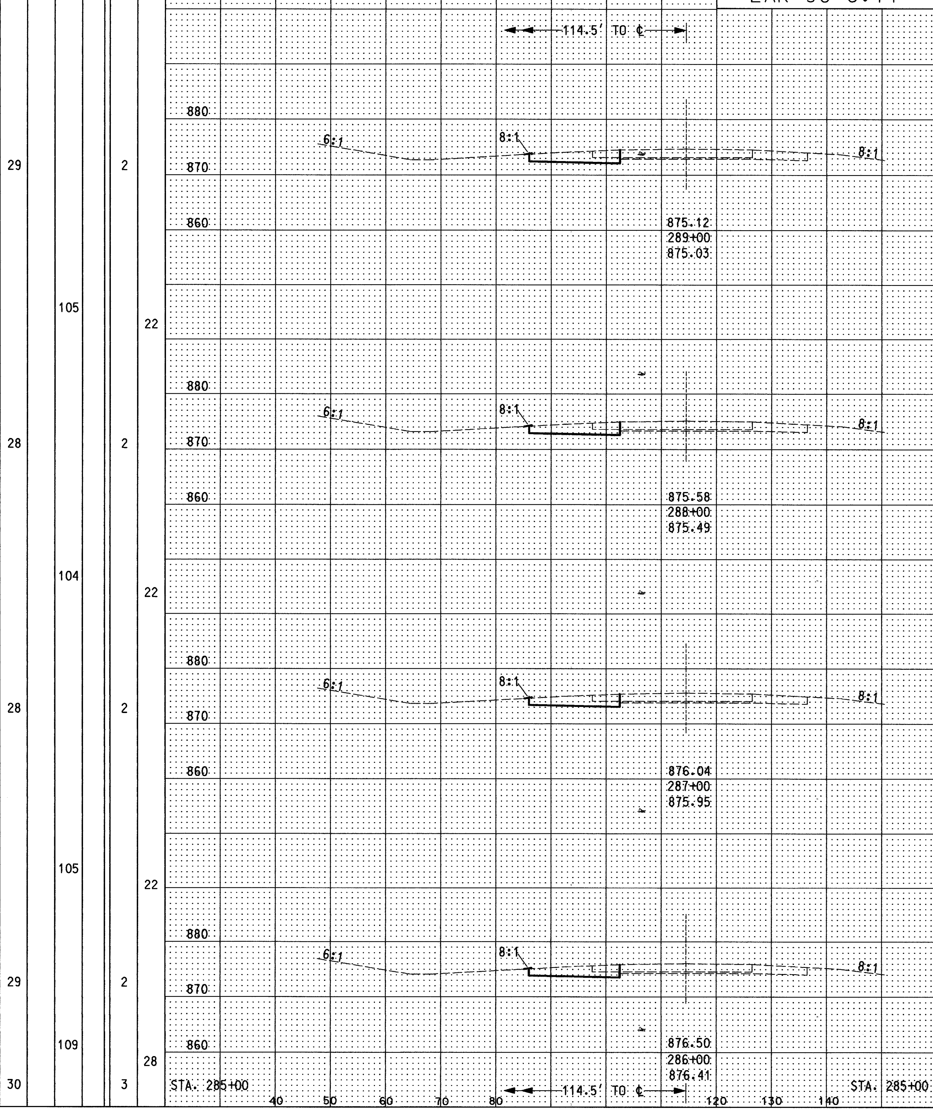
CROSS SECTION STA. 286+00 TO STA. 289+00 (WB) STA. 286+00 TO STA. 289+00 (EB)
