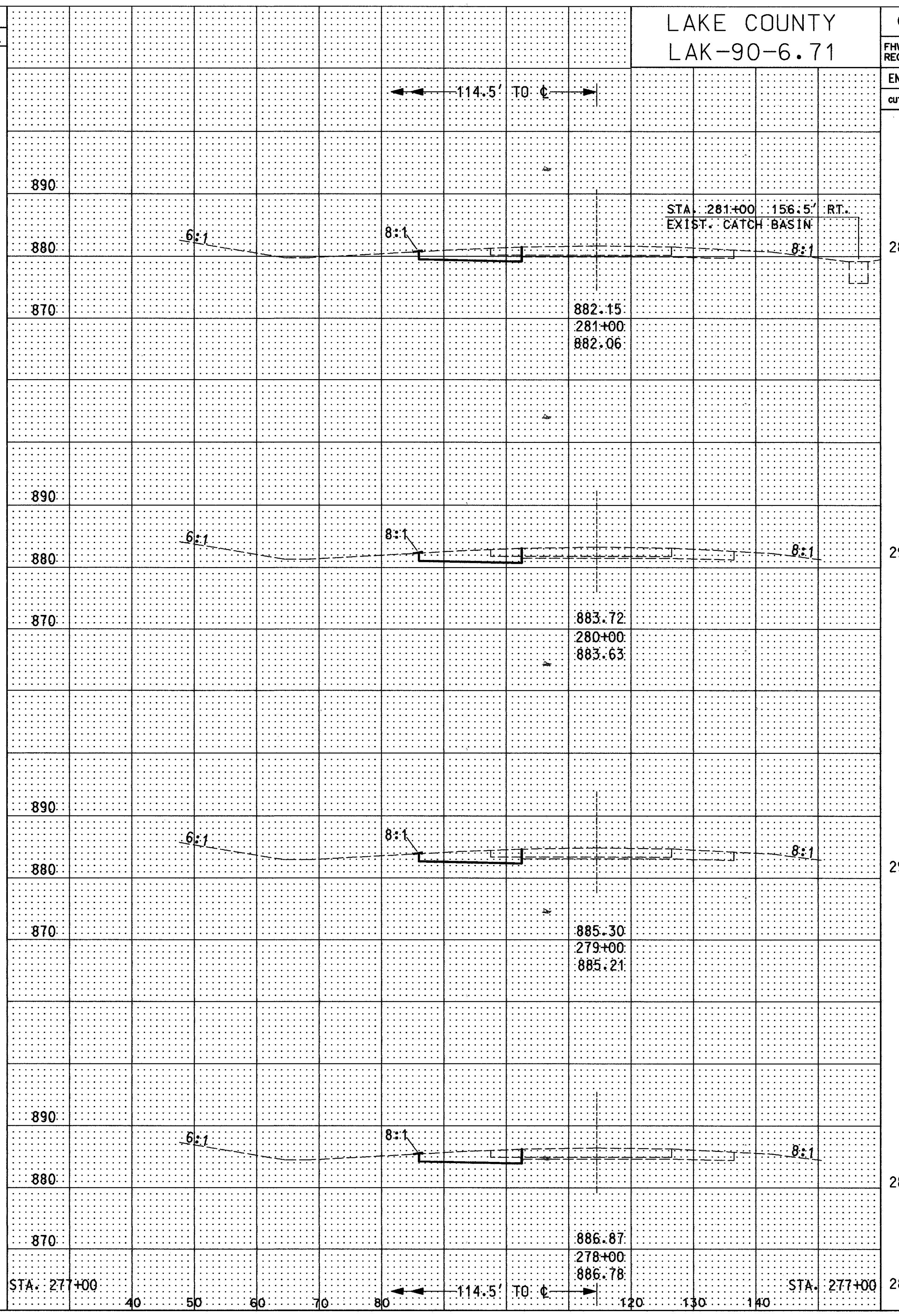
CROSS SECTION STA. 278+00 TO STA. 281+00 (WB) STA. 278+00 TO STA. 281+00 (EB)
