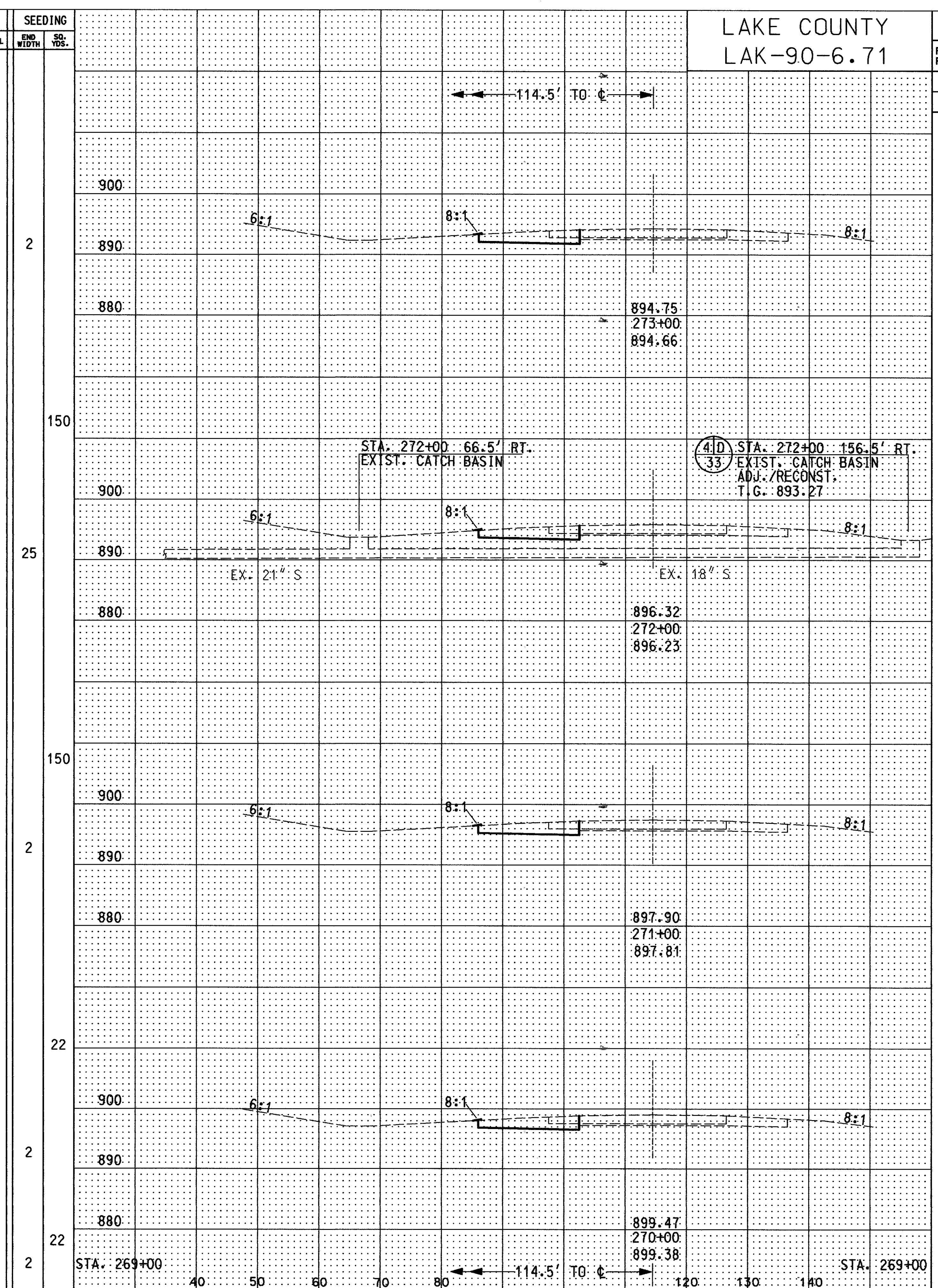
CROSS SECTION STA. 270+00 TO STA. 273+00 (WB) STA. 270+00 TO STA. 273+00 (EB)
