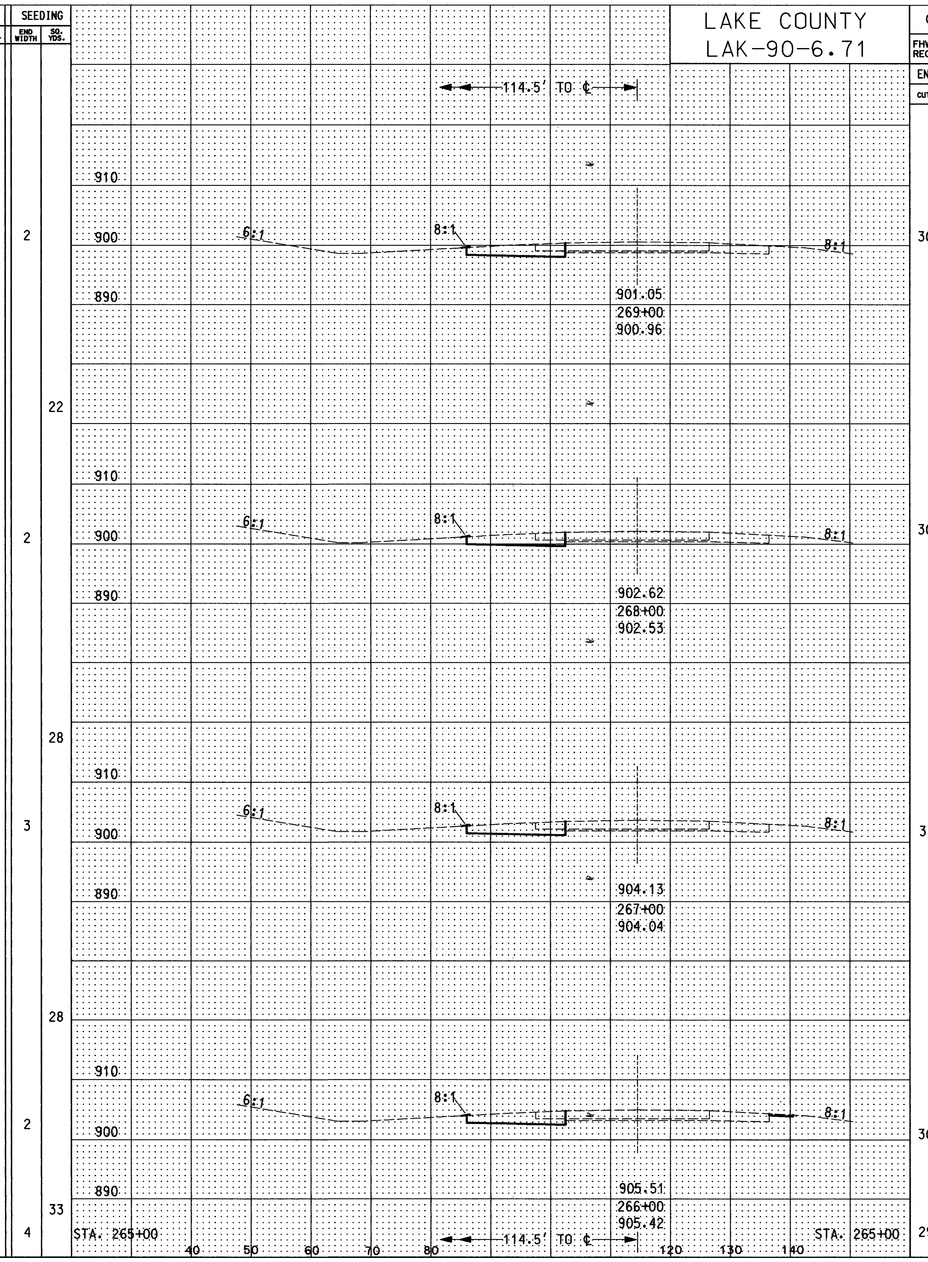
CROSS SECTION STA. 266+00 TO STA. 269+00 (WB) STA. 266+00 TO STA. 269+00 (EB)
