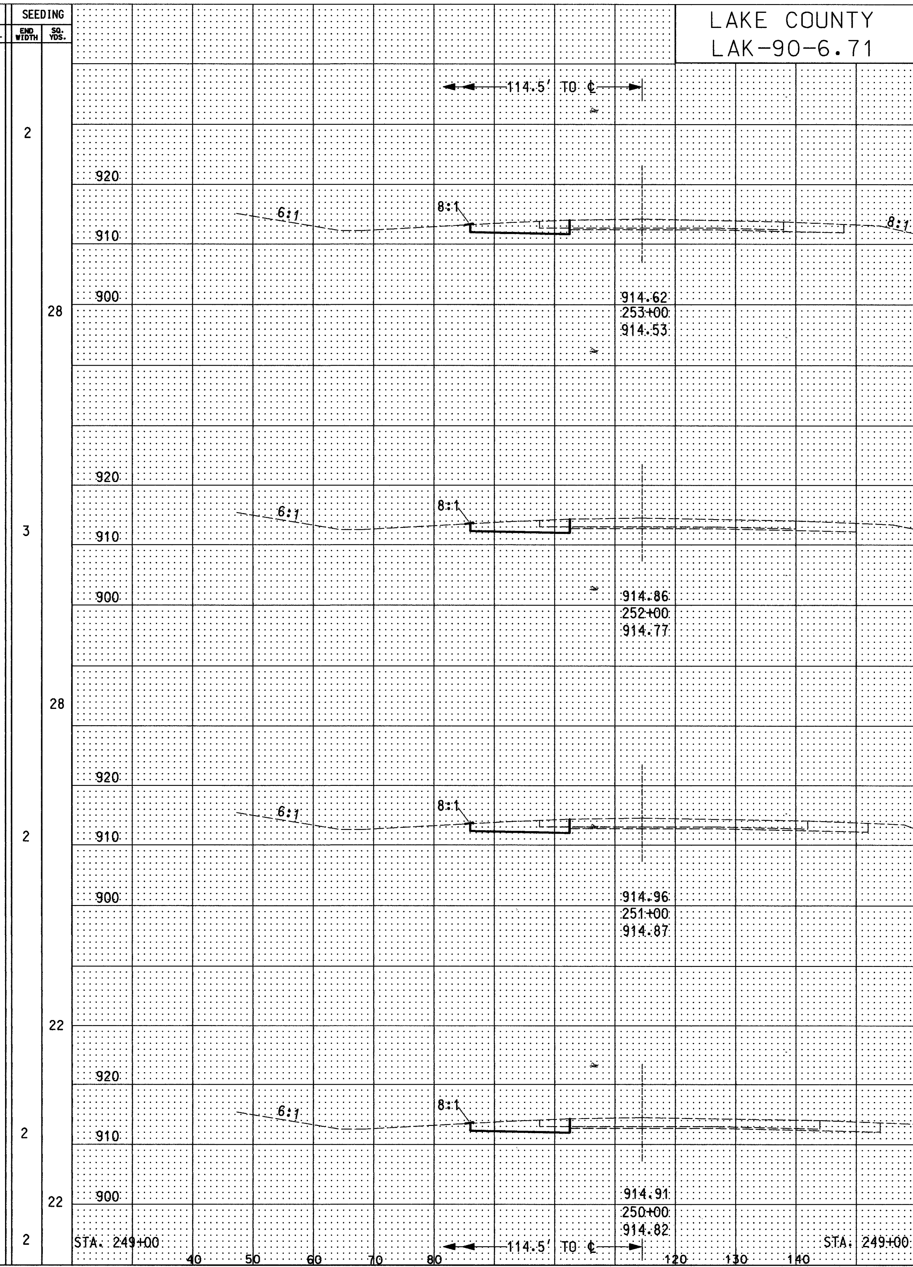
CROSS SECTION STA. 250+00 TO STA. 253+00 (WB) STA. 250+00 TO STA. 253+00 (EB)
