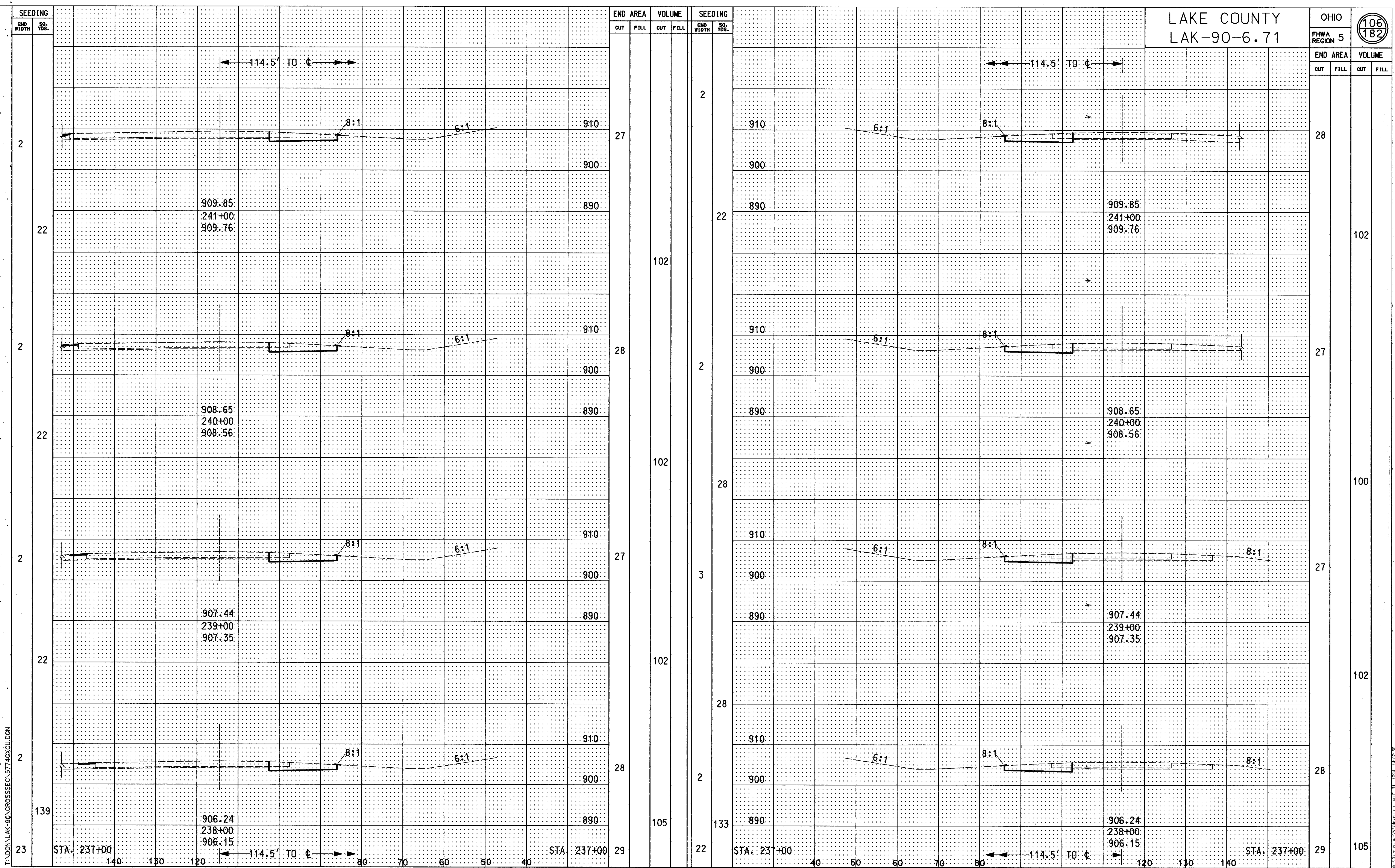
CROSS SECTION STA. 238+00 TO STA. 241+00 (WB) STA. 238+00 TO STA. 241+00 (EB)
