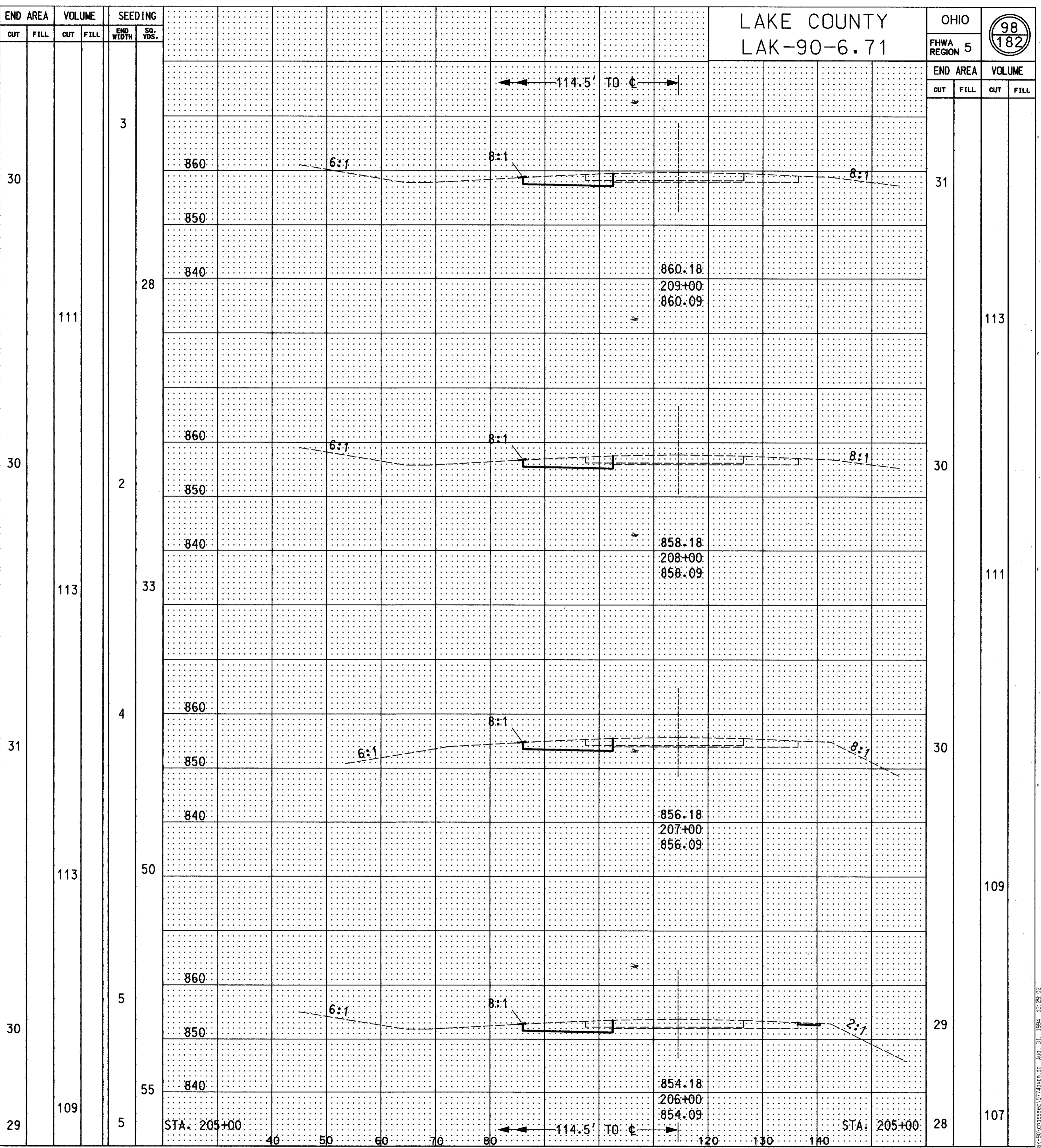
CROSS SECTION STA. 206+00 TO STA. 209+00 (WB) STA. 206+00 TO 209+00 (EB)
