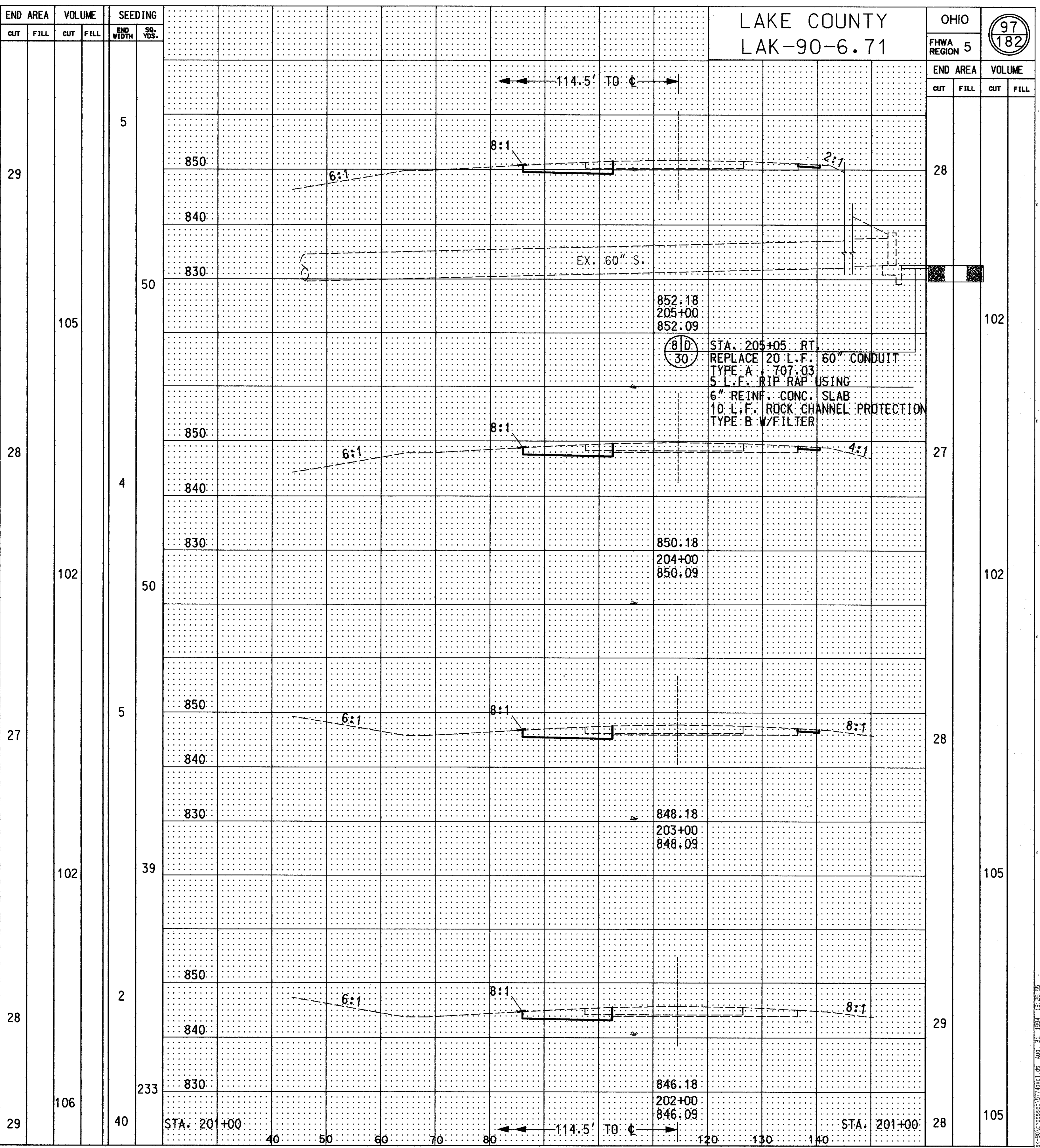
CROSS SECTION STA. 202+00 TO STA. 205+00 (WB) STA. 202+00 TO 205+00 (EB)
