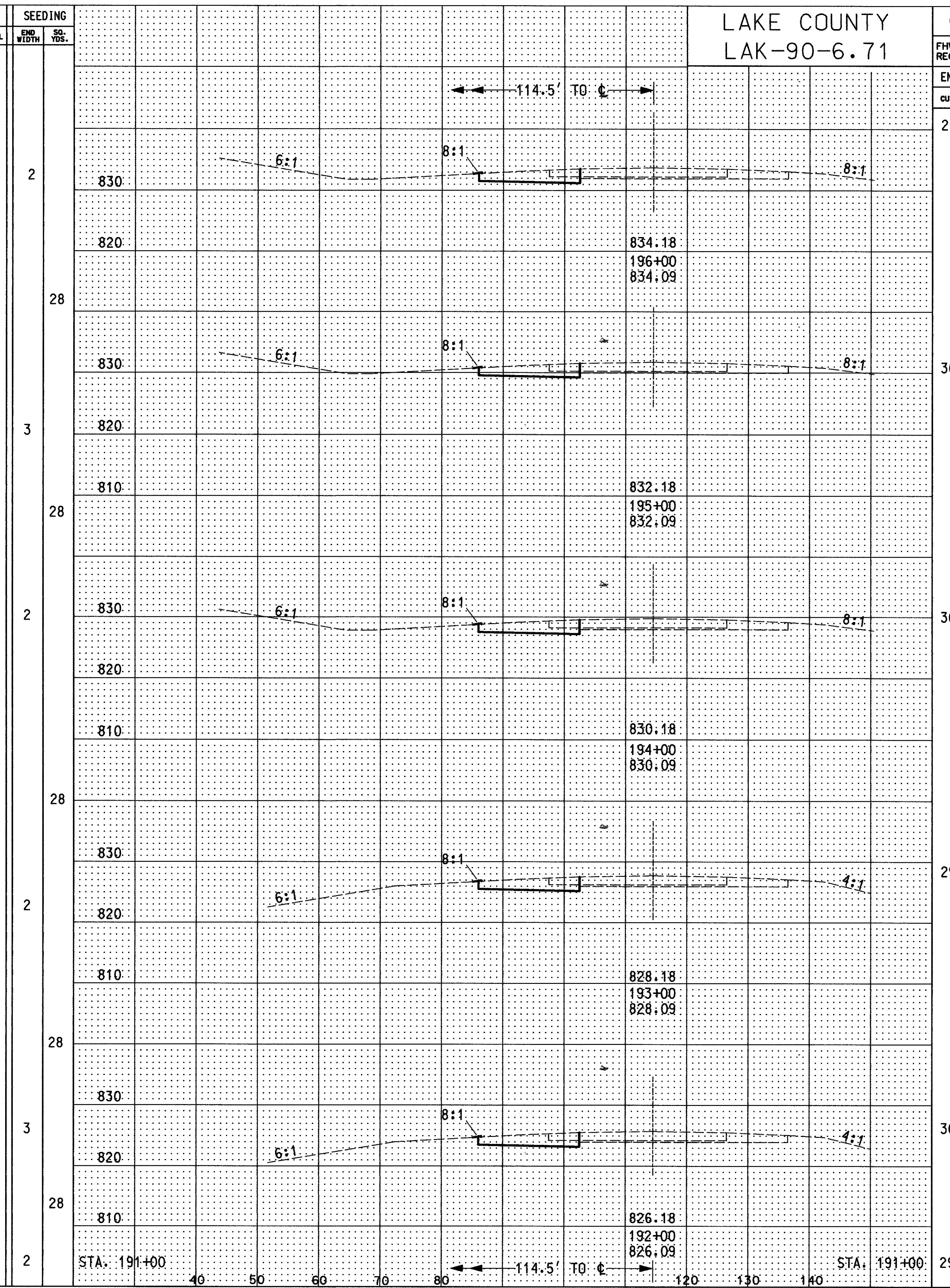
CROSS SECTION STA. 192+00 TO STA. 196+00 (WB) & STA. 192+00 TO STA. 196+00 (EB)
