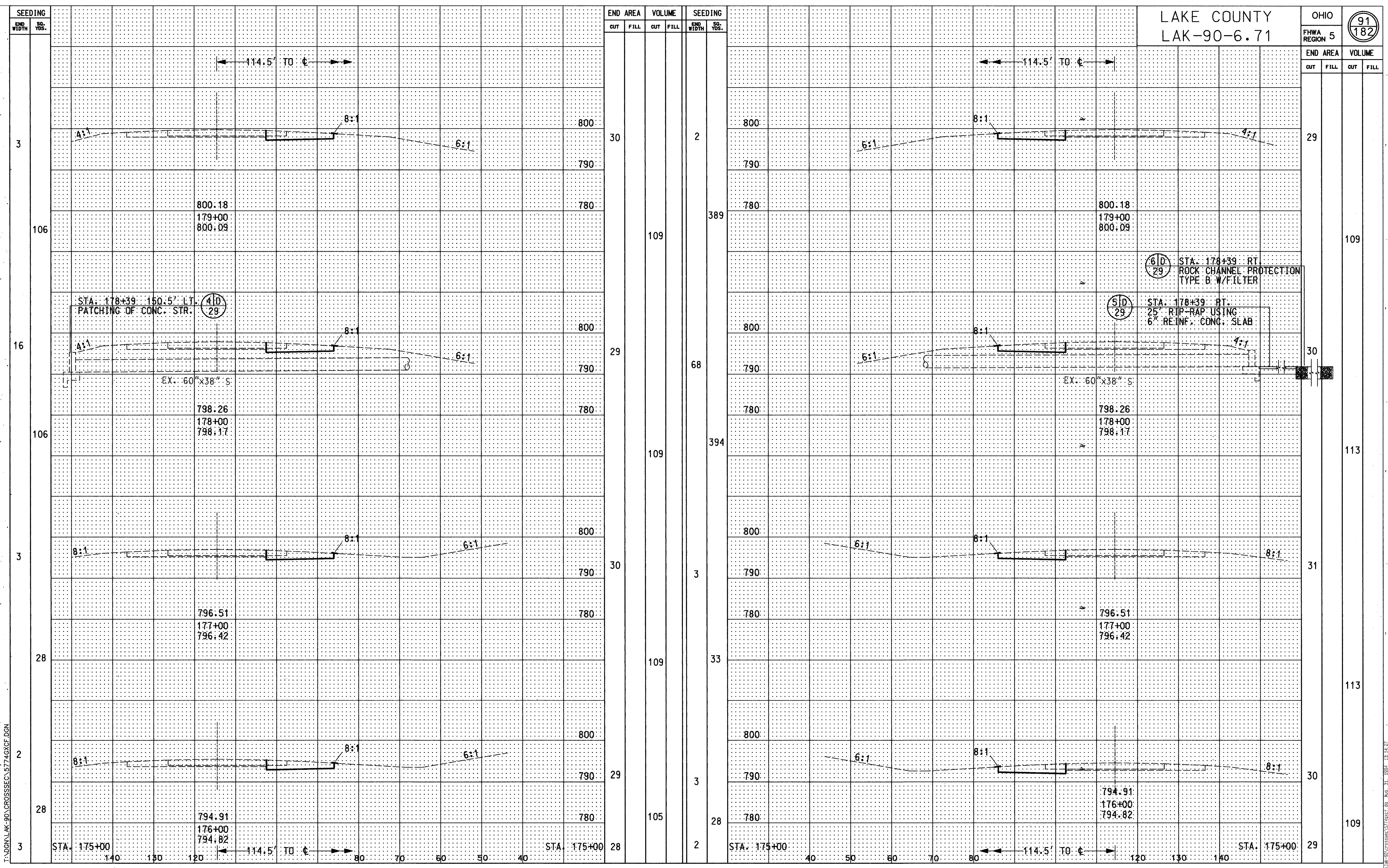
CROSS SECTION STA. 176+00 TO STA. 179+00 (WB) & STA. 176+00 TO STA. 179+00 (EB)
