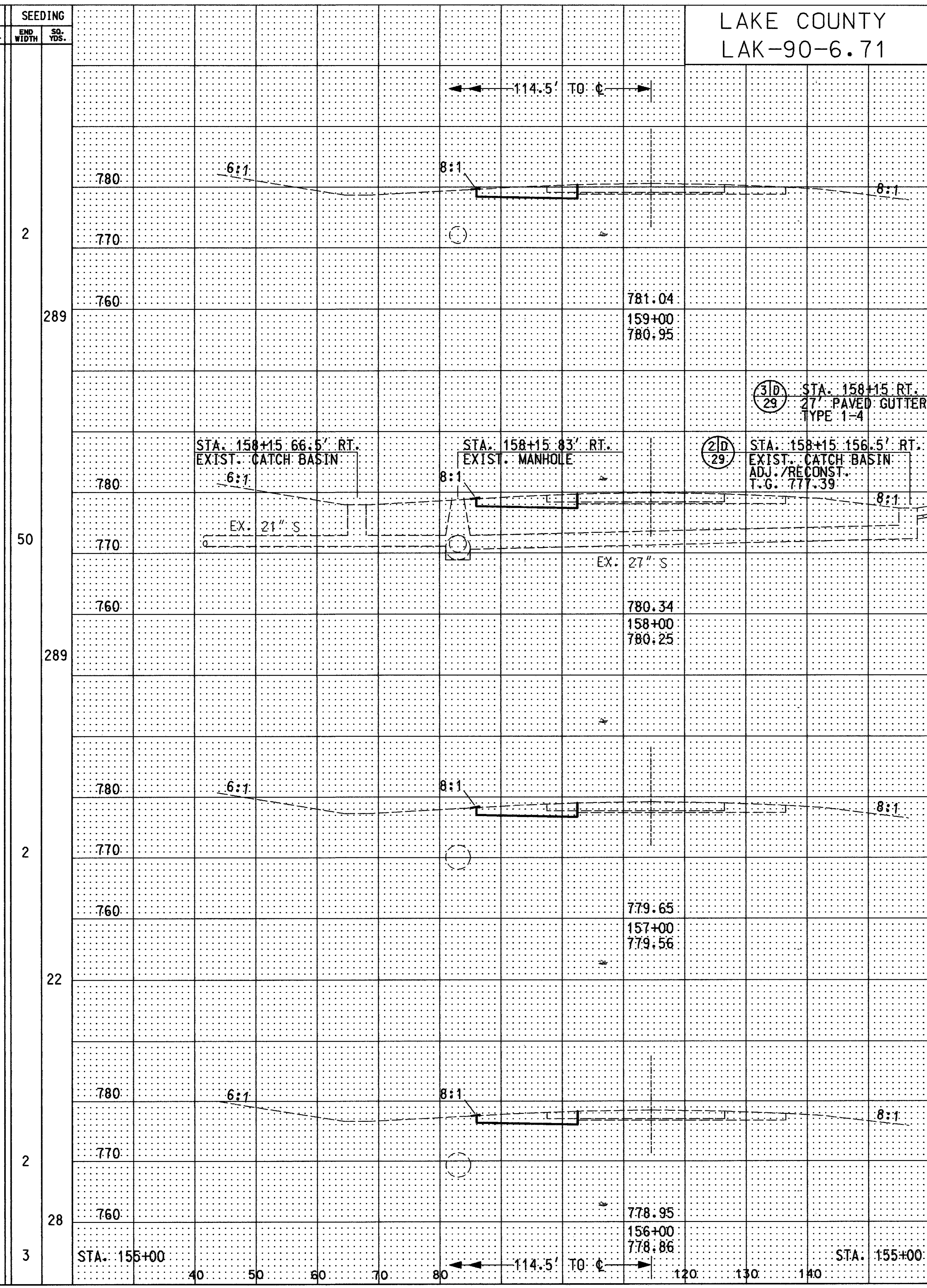
CROSS SECTION STA. 156+00 TO STA. 159+00 (WB) & STA. 156+00 TO STA. 159+00 (EB)
