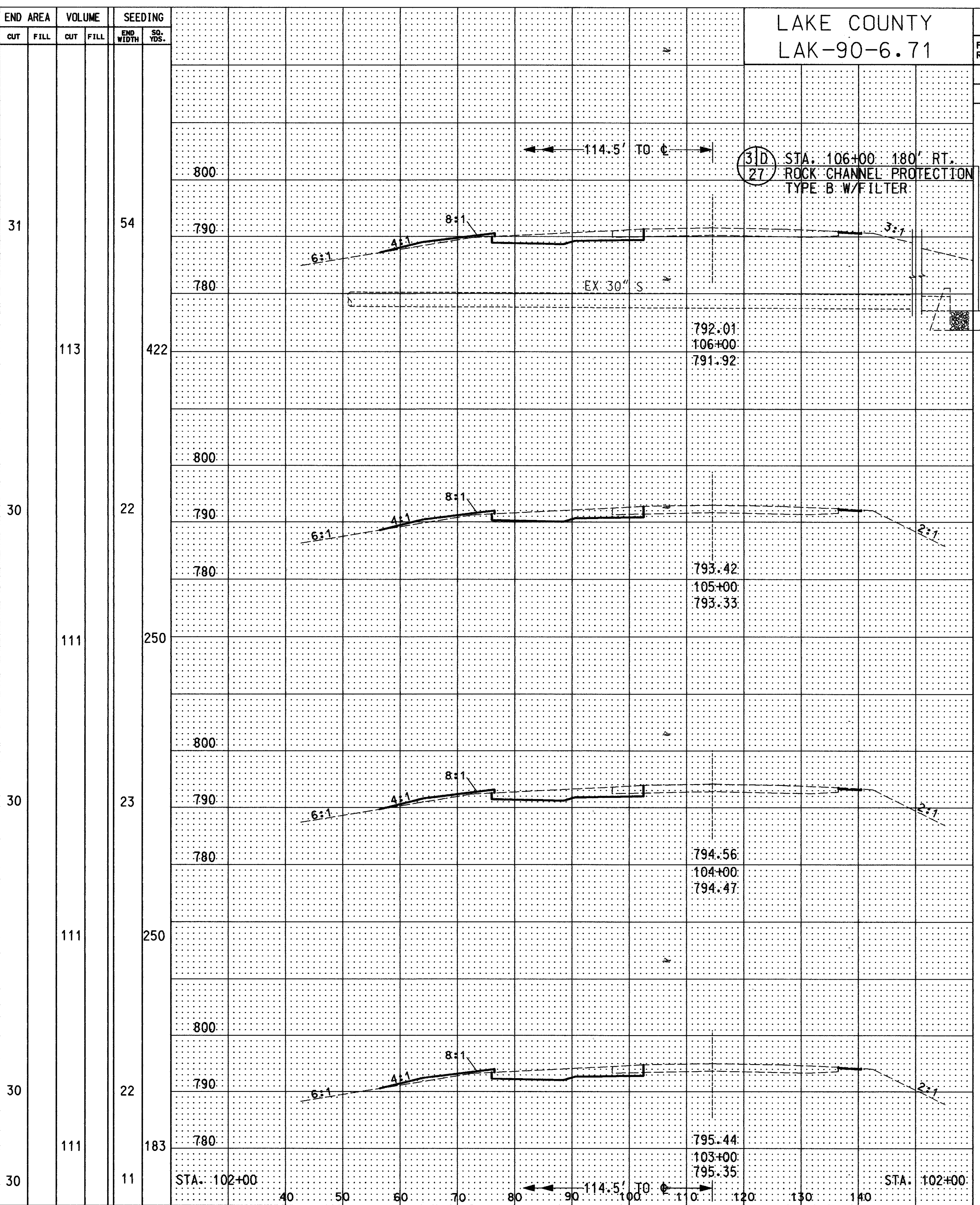
CROSS SECTION STA. 103+00 TO STA. 106+00 (WB) STA. 103+00 TO STA. 106+00 (EB)
