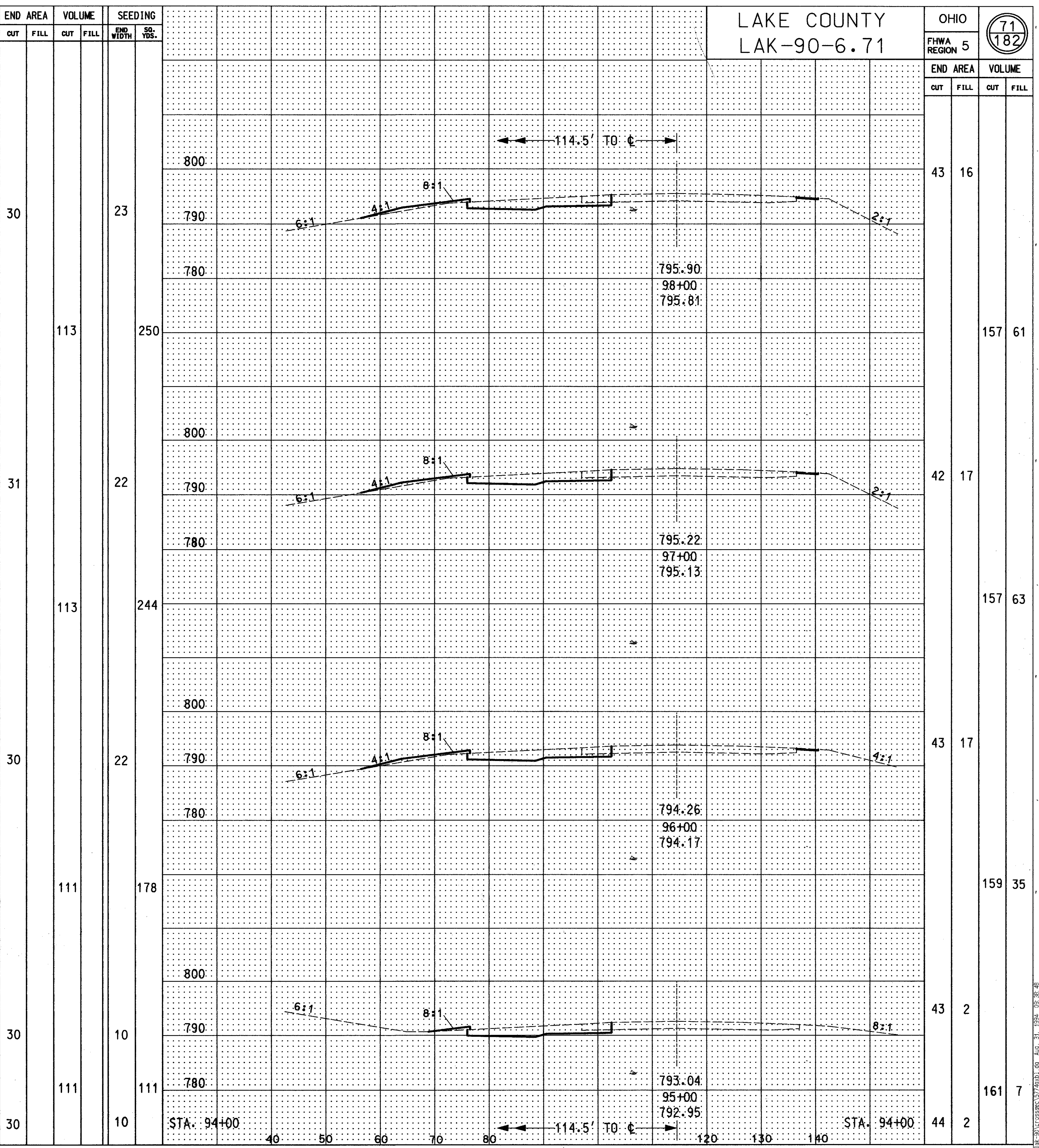
CROSS SECTION STA. 95+00 TO STA. 98+00 (WB) STA. 95+00 TO STA. 98+00 (EB)
