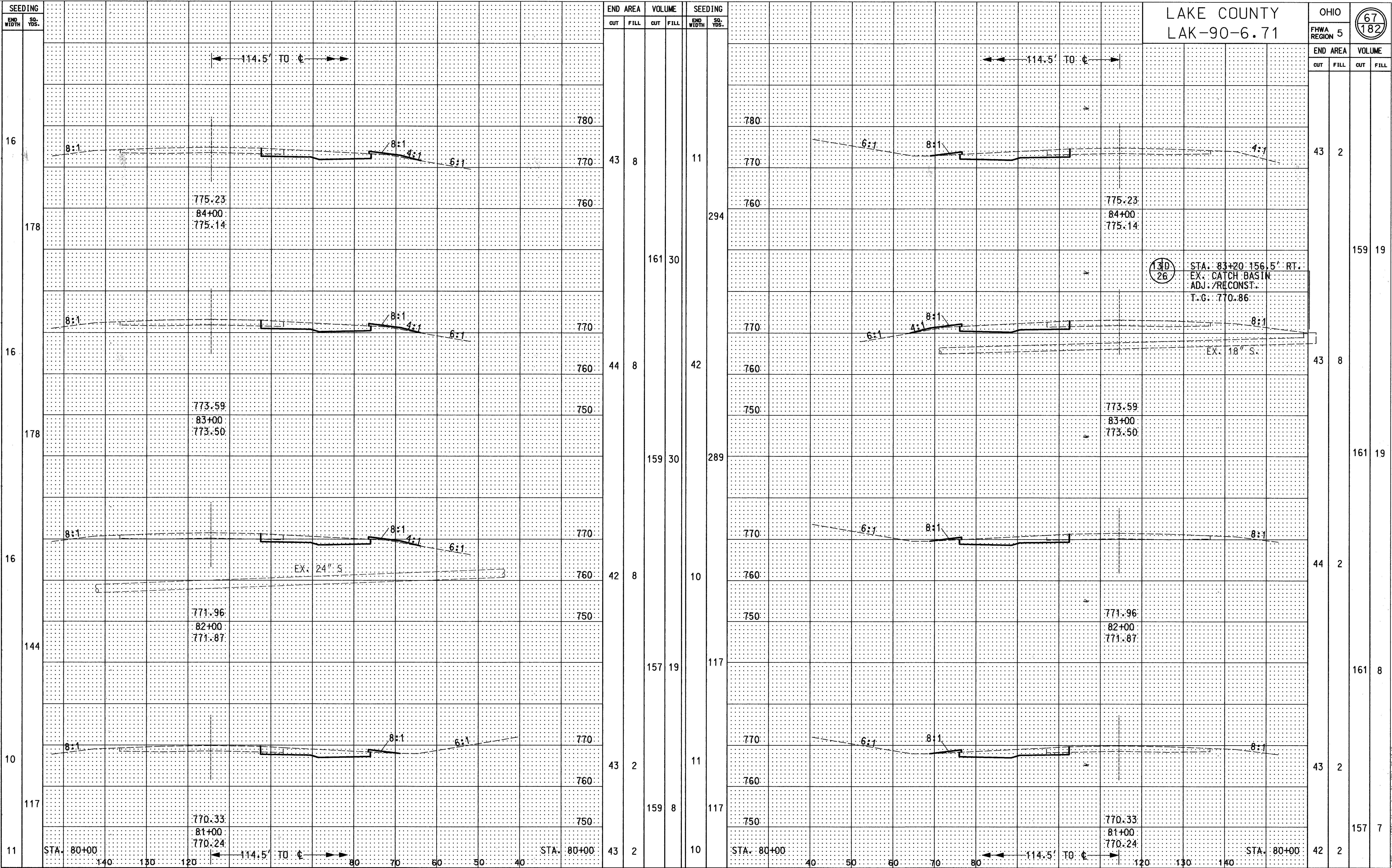
CROSS SECTION STA. 81+00 TO STA. 84+00 (WB) STA. 81+00 TO STA. 84+00 (EB)
