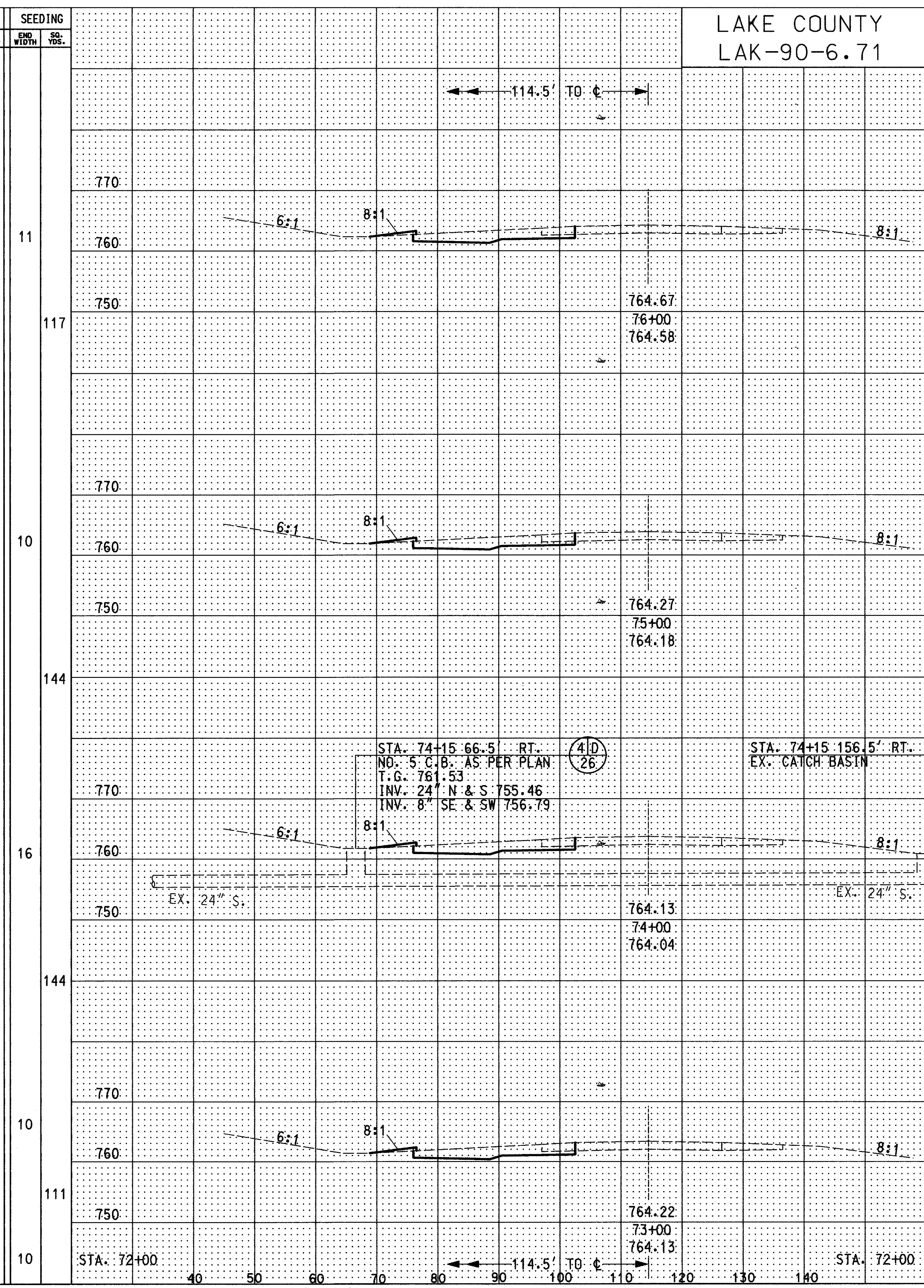
CROSS SECTION STA. 73+00 TO STA. 76+00 (WB) STA. 73+00 TO STA. 76+00 (EB)
