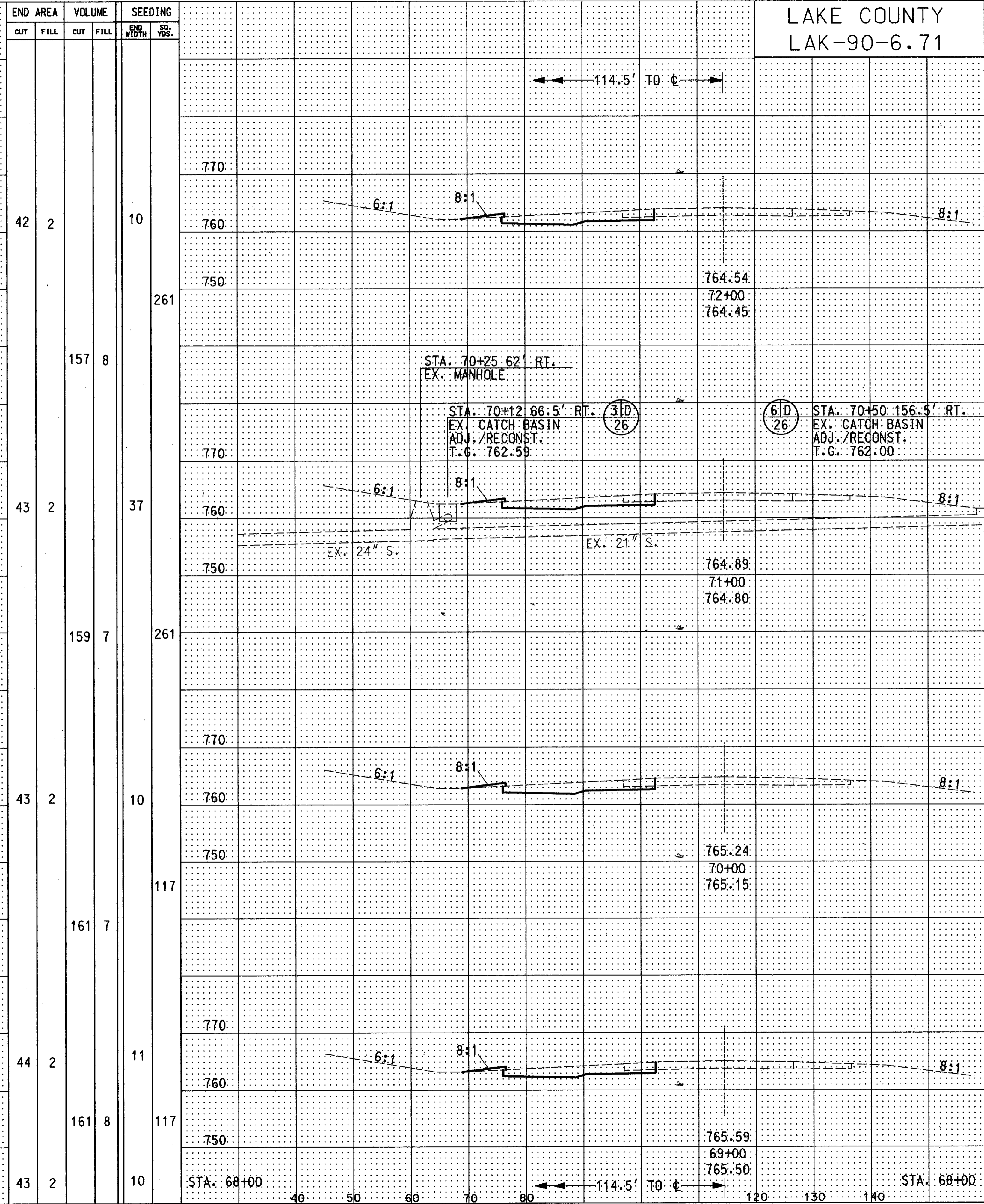
CROSS SECTION STA. 69+00 TO STA. 72+00 (WB) STA. 69+00 TO STA. 72+00 (EB)
