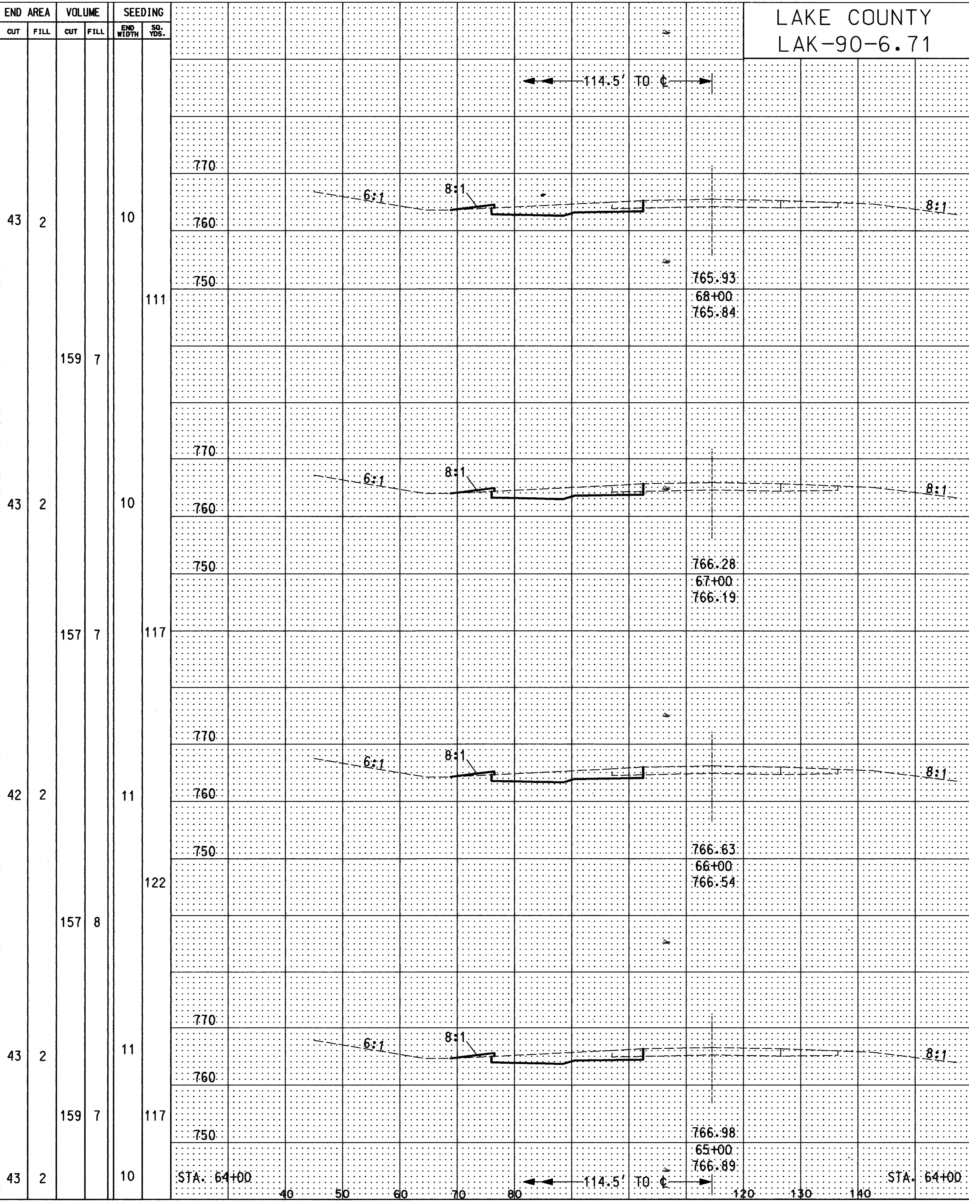
CROSS SECTION STA. 65+00 TO STA. 68+00 (WB) STA. 65+00 TO STA. 68+00 (EB)
