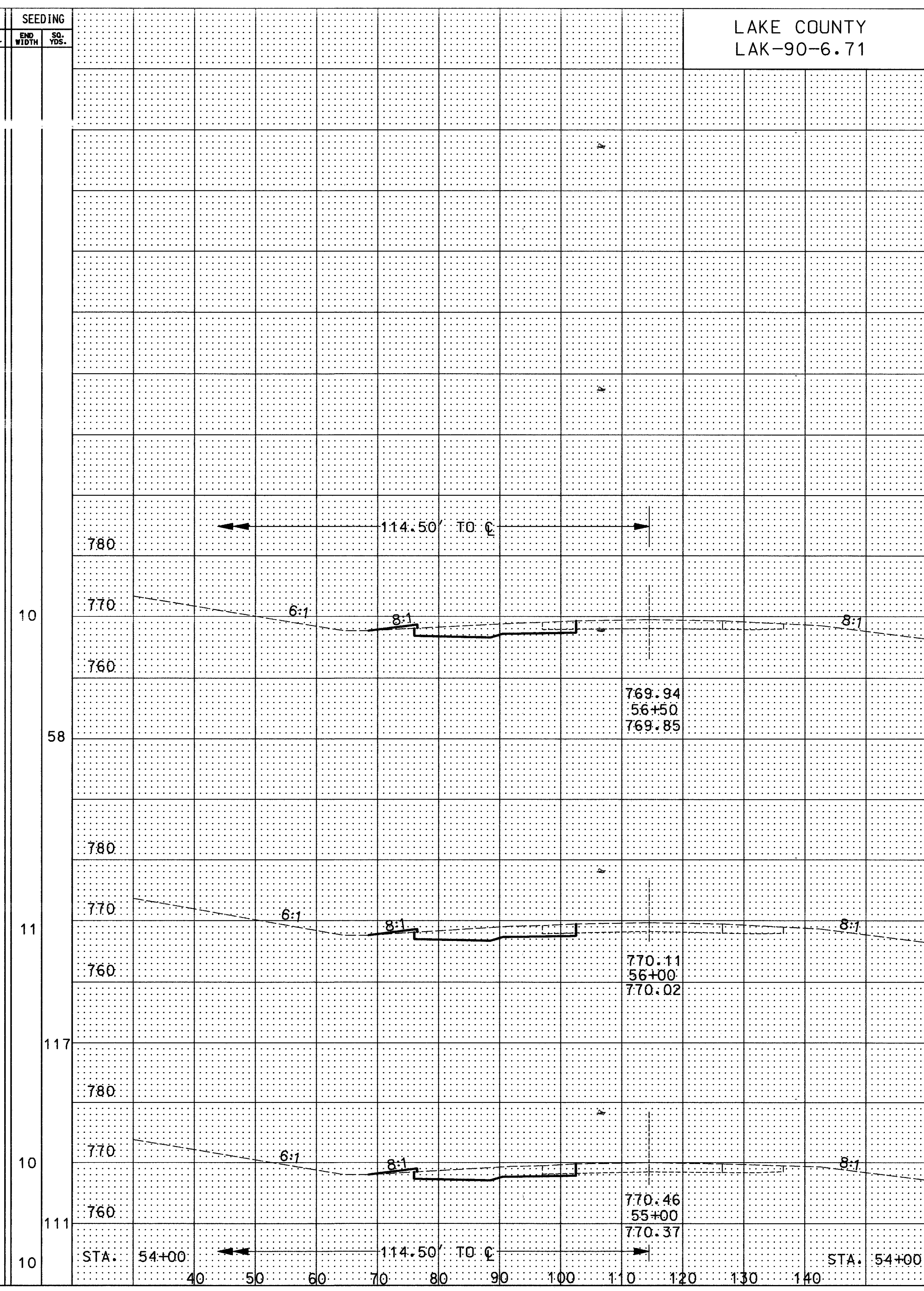
CROSS SECTIONS STA. 55+00 TO STA. 56+50 (WB) & STA. 55+00 TO STA. 56+50 (EB)
