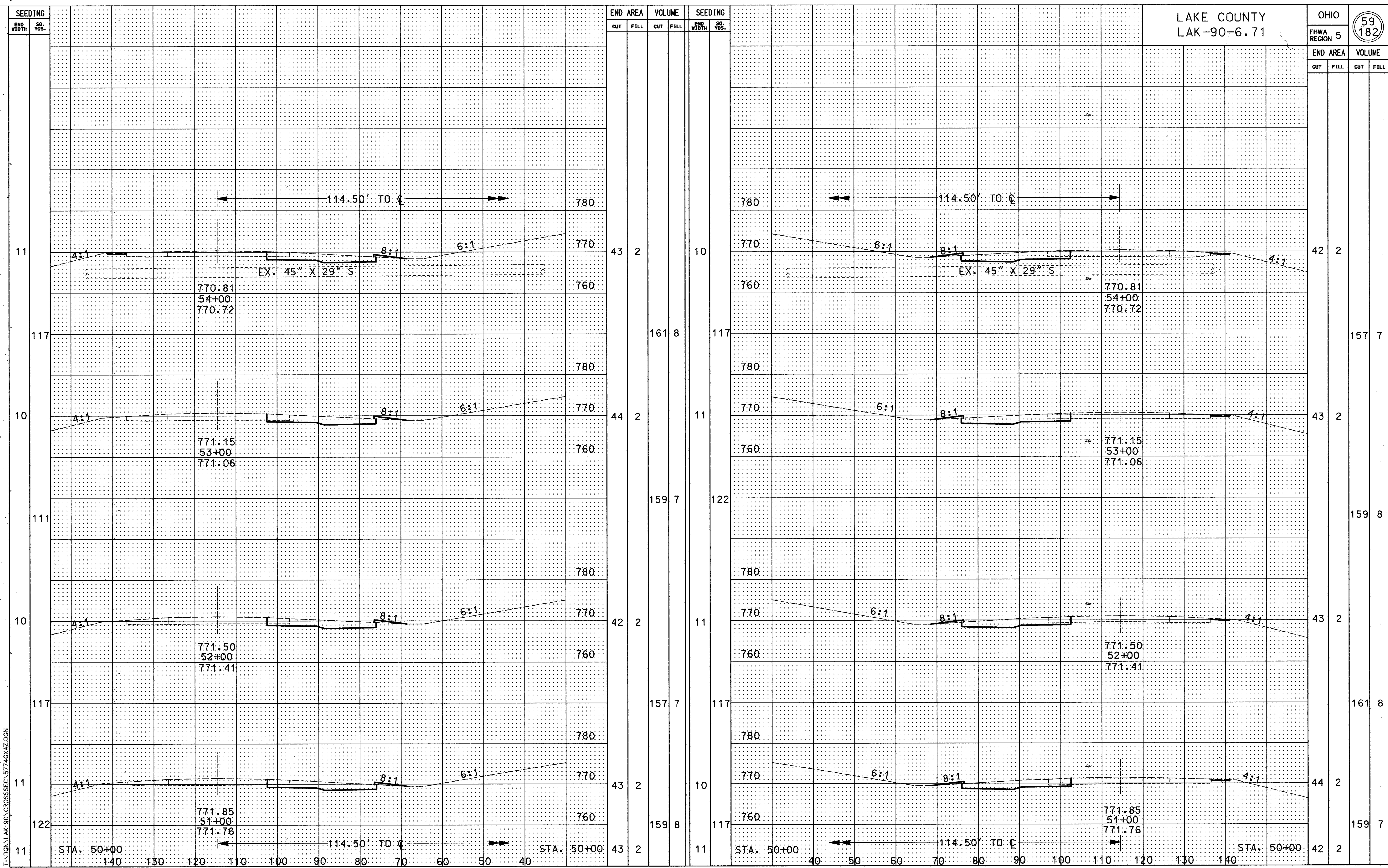
CROSS SECTIONS STA. 51+00 TO STA. 54+00 (WB) & STA. 51+00 TO STA. 54+00 (EB)
